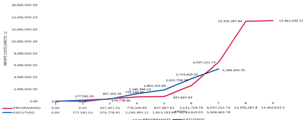
CURVA "S" - VALORIZACION DE OBRA N° 06
