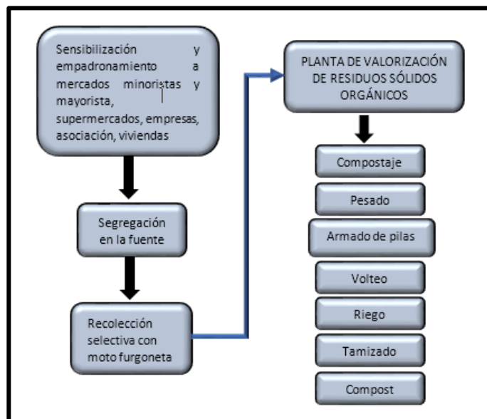
Ilustración N° 4. Flujo del proceso de valorización de residuos sólidos orgánicos
