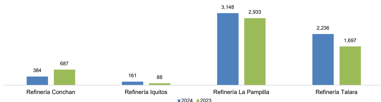
Producción de combustibles por refinería (MBLS), abril 2024-2023
