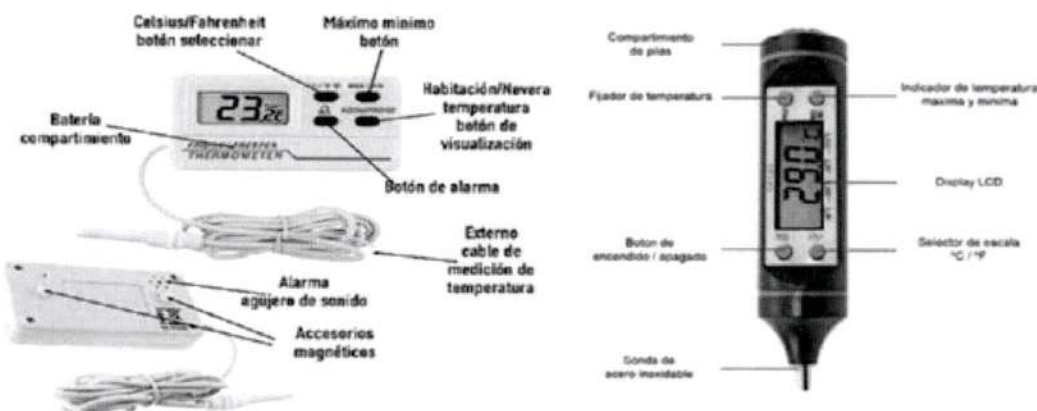
Imagen 01. Partes del termómetro digital LCD para refrigerador y congelador.
