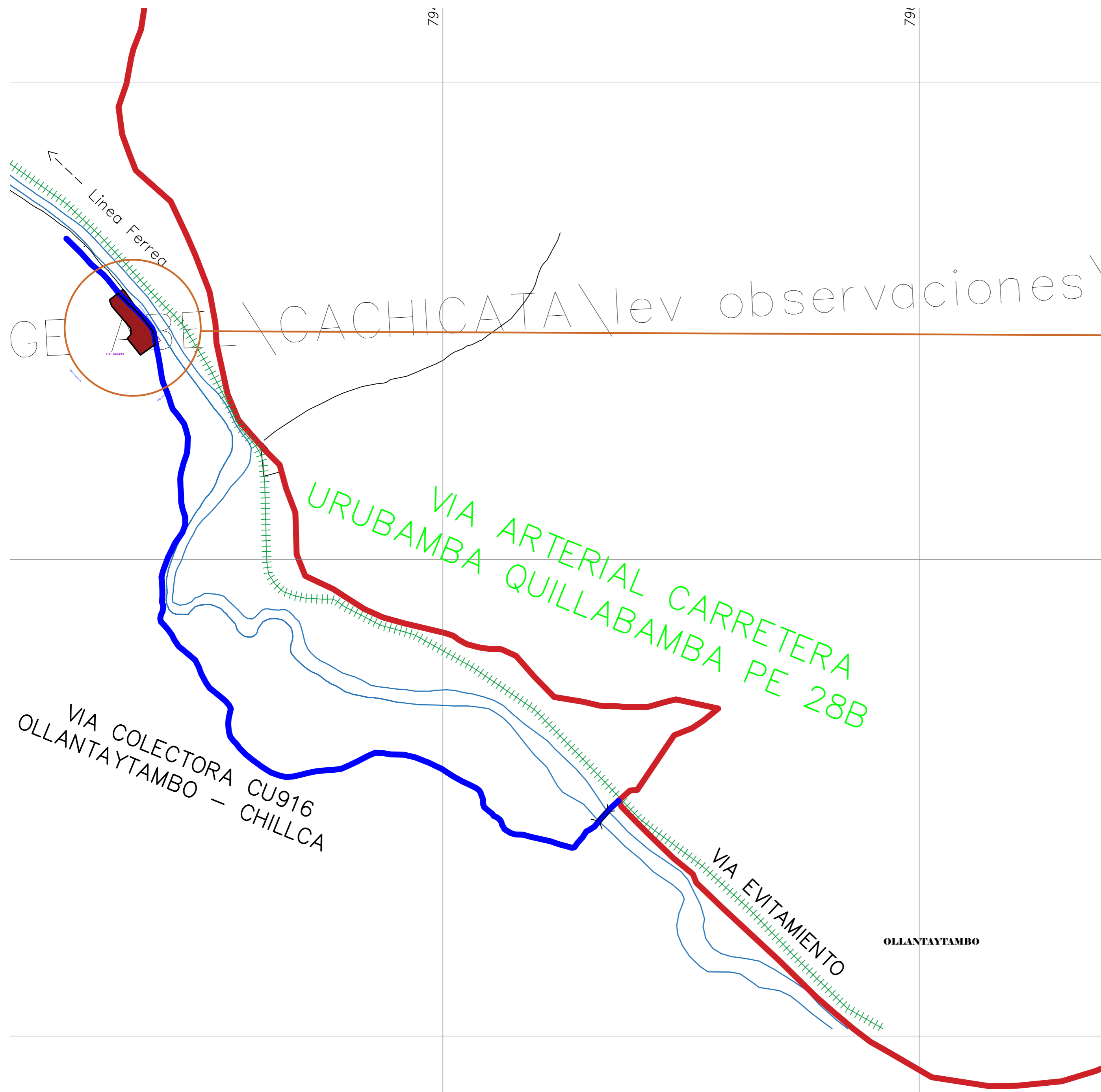
PLANO DE INTEGRACION VIAL ESC. 1/2500
