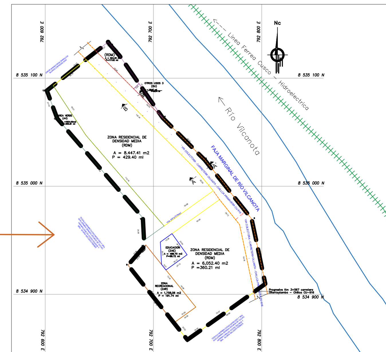
PLANO DE UBICACION ESC. 1/2000
