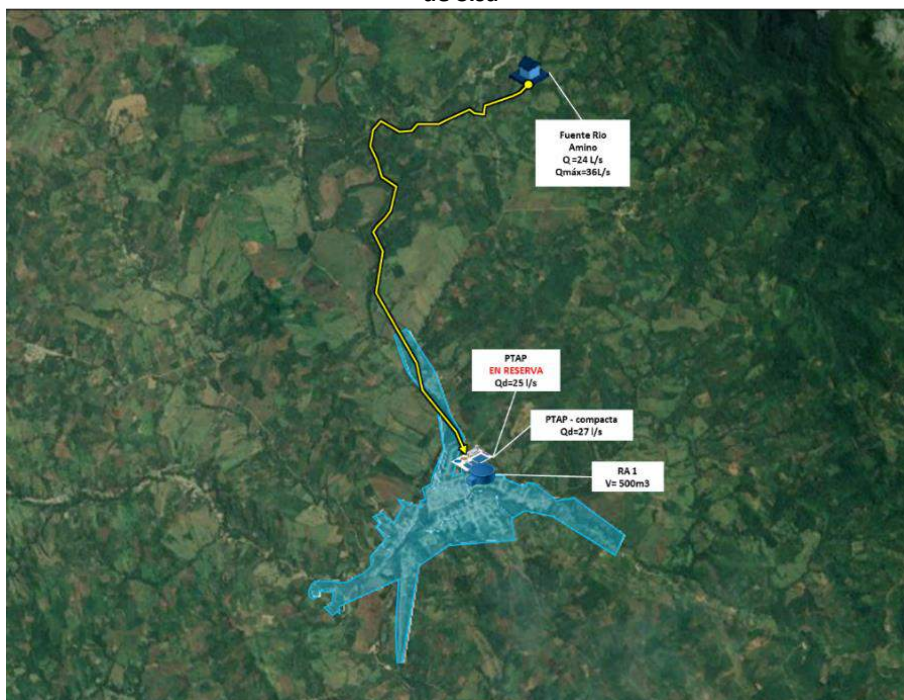
Imagen N° 50: Esquema general del sistema de abastecimiento de agua potable – Localidad San José de Sisa
