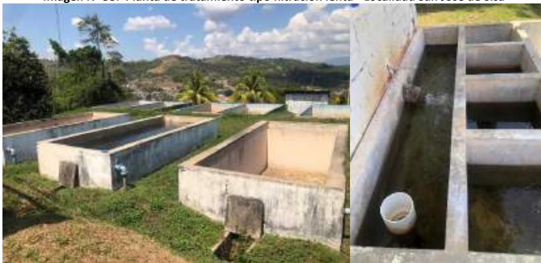
Imagen N° 53: Planta de tratamiento tipo filtración lenta - Localidad San José de Sisa
