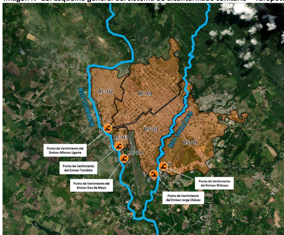
Imagen N° 28: Esquema general del sistema de alcantarillado sanitario – Tarapoto
