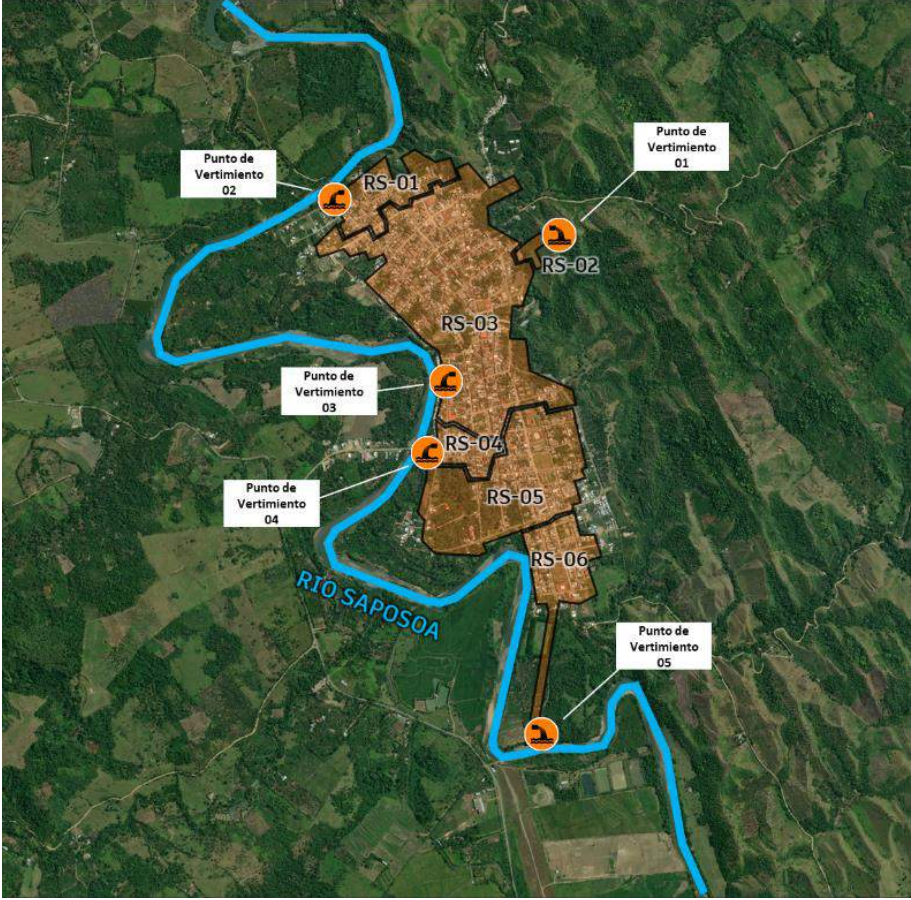
Imagen N° 38: Esquema general del sistema de alcantarillado sanitario – Localidad Saposoa
