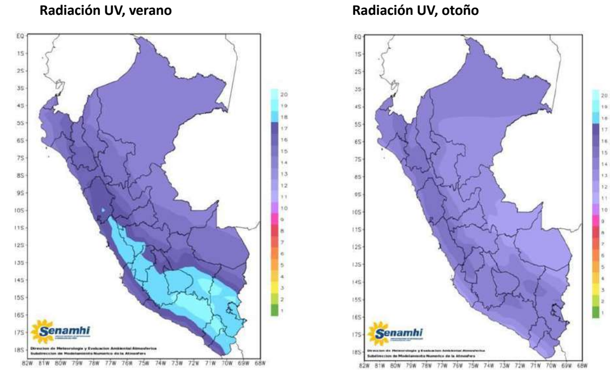
Figura 47. Radiación UV estacional sin nubosidad, 1995-2003
