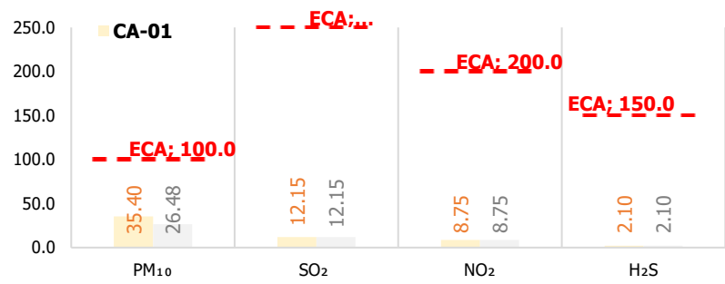
Figura 62. Monitoreo de calidad del aire, Bellavista 2022
