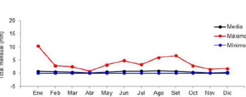
Figura 43. Comportamiento de la precipitación acumulada mensual, 1970-2021
