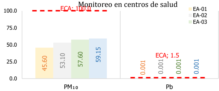
Figura 66. Monitoreo de calidad del aire, Ventanilla 2019
