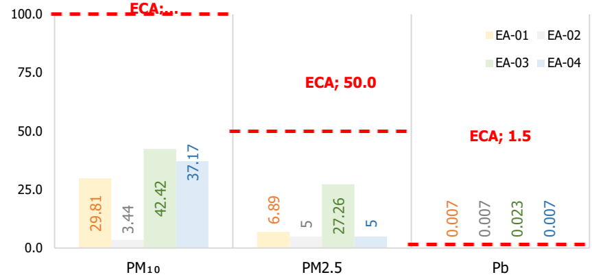
Figura 68. Monitoreo de calidad del aire, Callao 2019
