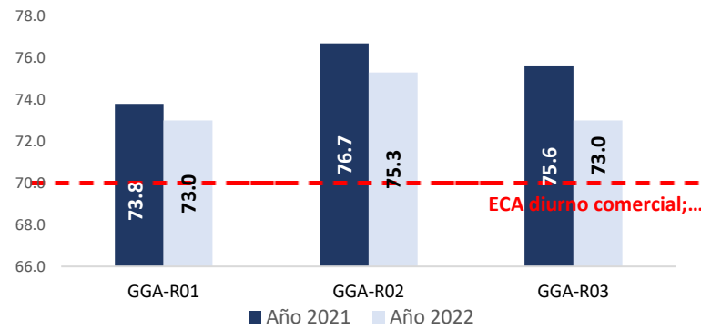
Figura 71. Monitoreo de calidad del ruido, La Perla 2022
