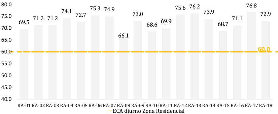
Figura 70. Monitoreo de calidad del ruido, Bellavista 2022
