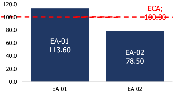
Figura 64. Monitoreo de calidad del aire, Mi Perú 2021
