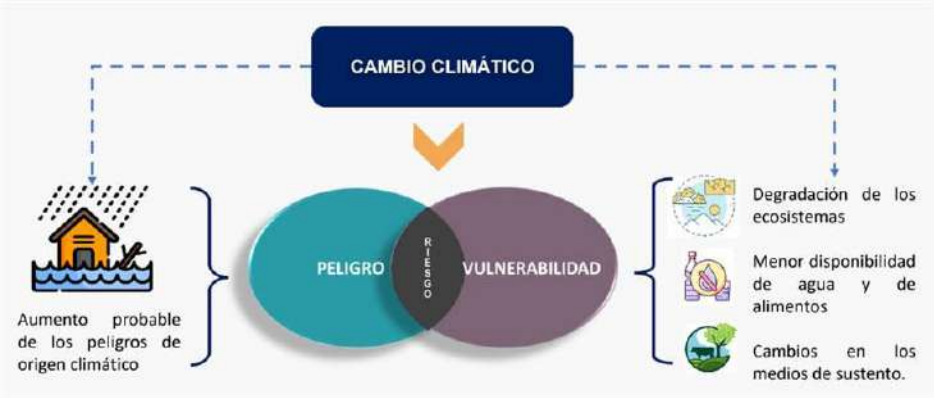
Figura 173. Efectos del cambio climático en la gestión del riesgo de desastres
