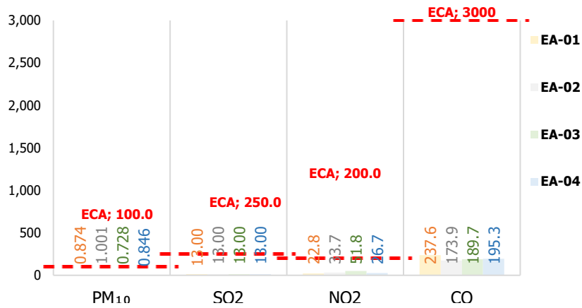
Figura 69. Monitoreo de calidad del aire, Carmen de la Legua 2021
