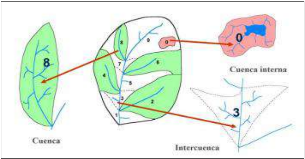
Figura 49. Clasificación de cuenca, Inter cuenca y cuenca interna
