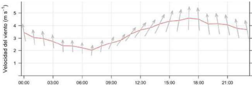
Figura 45. Comportamiento de la dirección y velocidad del viento, 1990-2020
