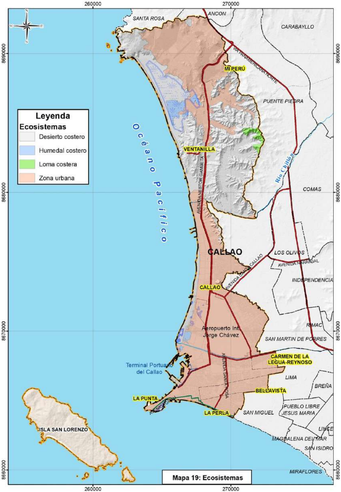
Mapa 19. Mapa de ecosistemas, Provincia Constitucional del Callao
