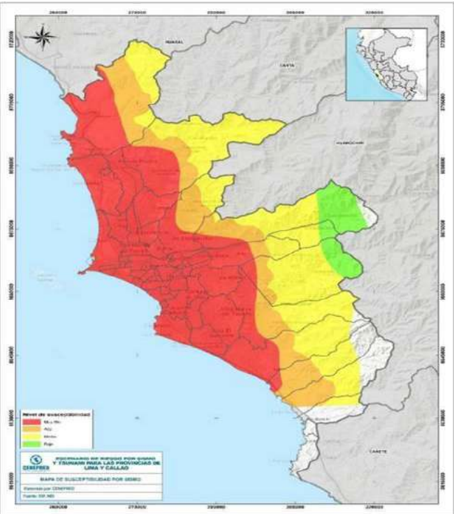
Figura 175. Mapa de susceptibilidad por sismo para las provincias de Lima y Callao
