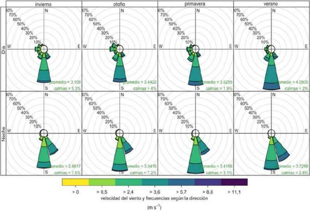
Figura 46. Rosa de viento estacional, 1990-2020
