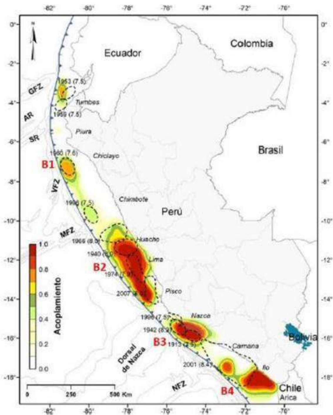
Figura 174. Distribución de las zonas de acoplamiento máximo en el borde costero del Perú
