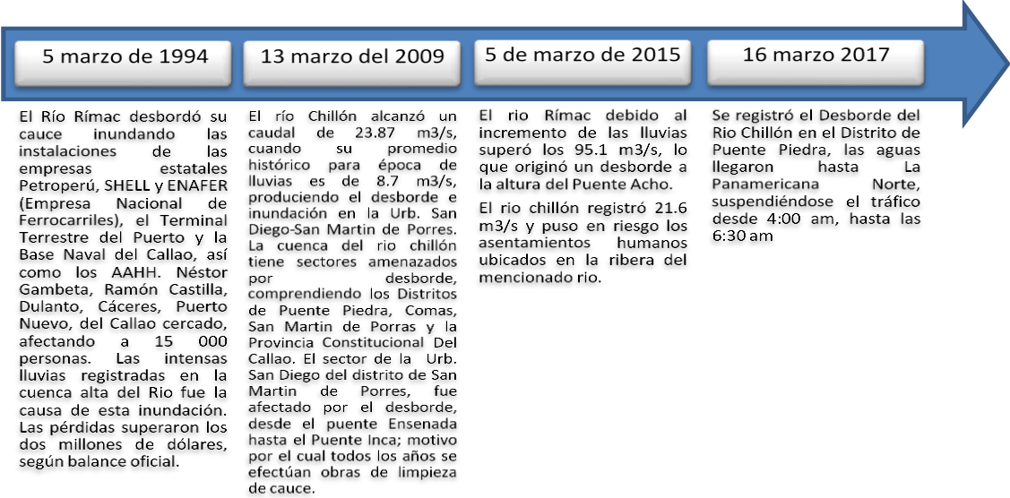
Figura 178. Eventos históricos de los Ríos Rímac y Chillón
