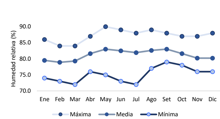
Figura 42. Comportamiento de la humedad relativa mensual, 1990-2020
