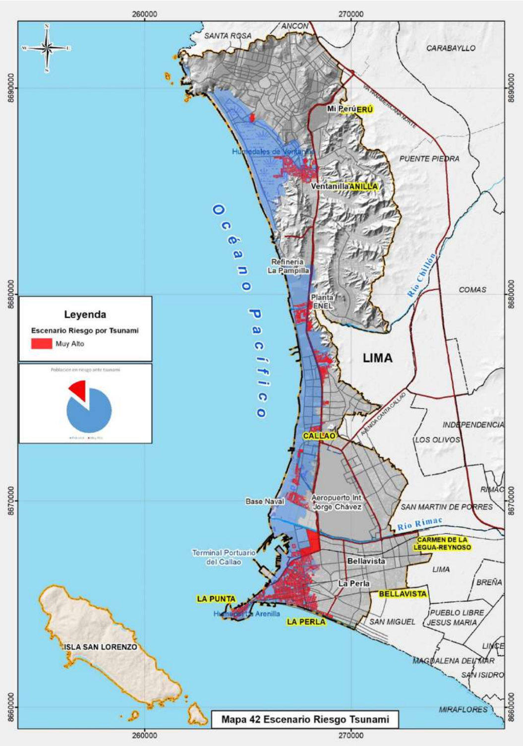
Mapa 43. Escenario de riesgo por tsunami en la Provincia Constitucional del Callao
