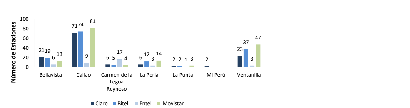
Figura 78. Distribución de estaciones base- 2017
