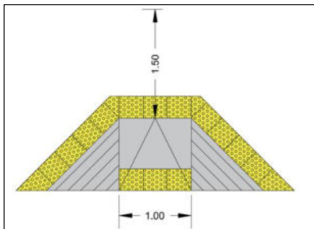
Figura 02. Rampa de tres planos
