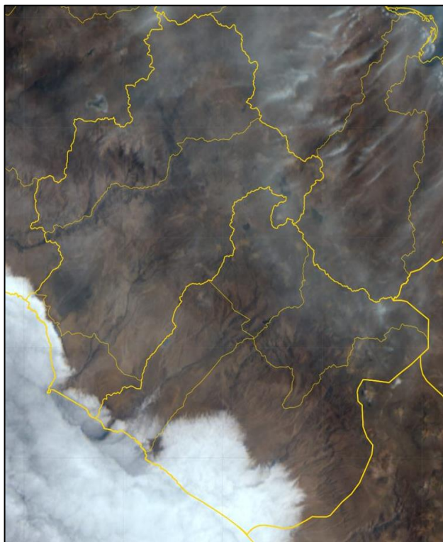
Fig1. Imagen satelital GOES 16 (06/11/2024 – 09 am)
