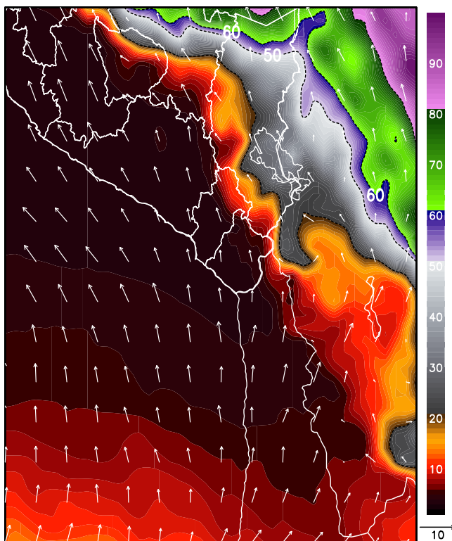
Fig2. Pronóstico de humedad relativa promedio (%) (500-300 hPa) (07/11/2024 – 07 am)
