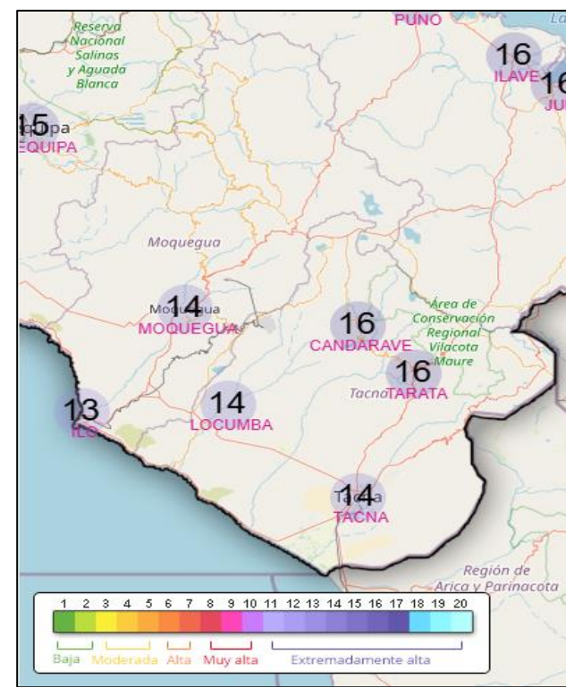
Fig3. Pronóstico de Índice de radiación ultravioleta máximo (IUV) (07/11/2024)
