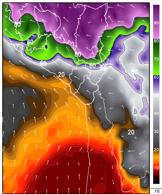
Fig2. Pronóstico de humedad relativa promedio (%) (500-300 hPa) (13/11/2024 – 07 am)
