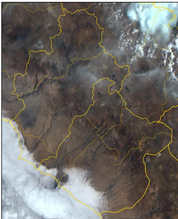
Fig1. Imagen satelital GOES 16 (12/11/2024 – 08:30 am)
