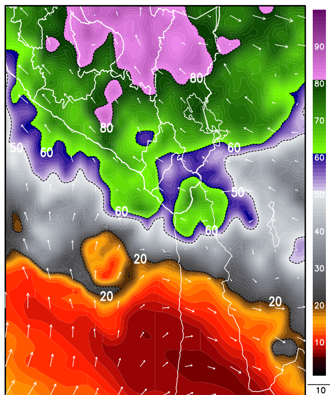
Fig2. Pronóstico de humedad relativa promedio (%) (500-300 hPa) (14/11/2024 – 07 am)
