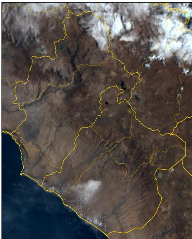
Fig1. Imagen satelital GOES 16 (13/11/2024 – 08:30 am)
