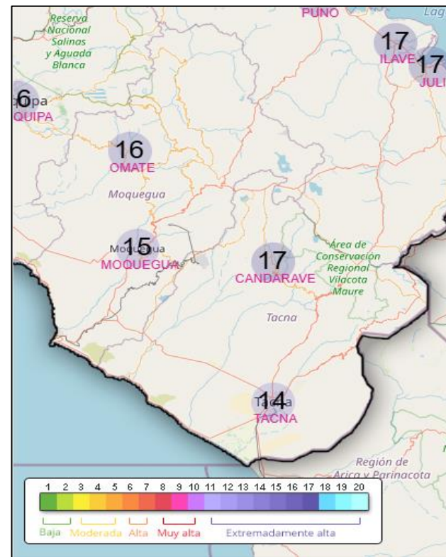
Fig3. Pronóstico de Índice de radiación ultravioleta máximo (IUV) (23/11/2024)
