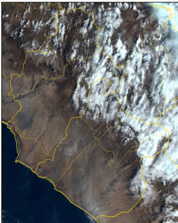
Fig1. Imagen satelital GOES 16 (22/11/2024 – 08:30 am)
