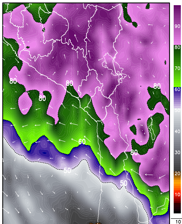
Fig2. Pronóstico de humedad relativa promedio (%) (500-300 hPa) (23/11/2024 – 01:00 pm)
