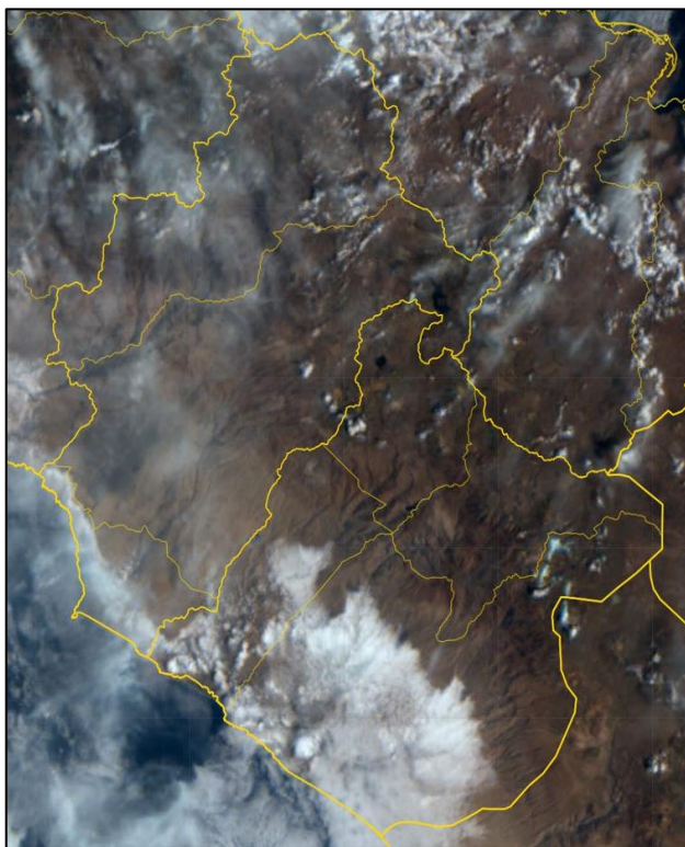
Fig1. Imagen satelital GOES 16 (27/11/2024 – 08:30 am)
