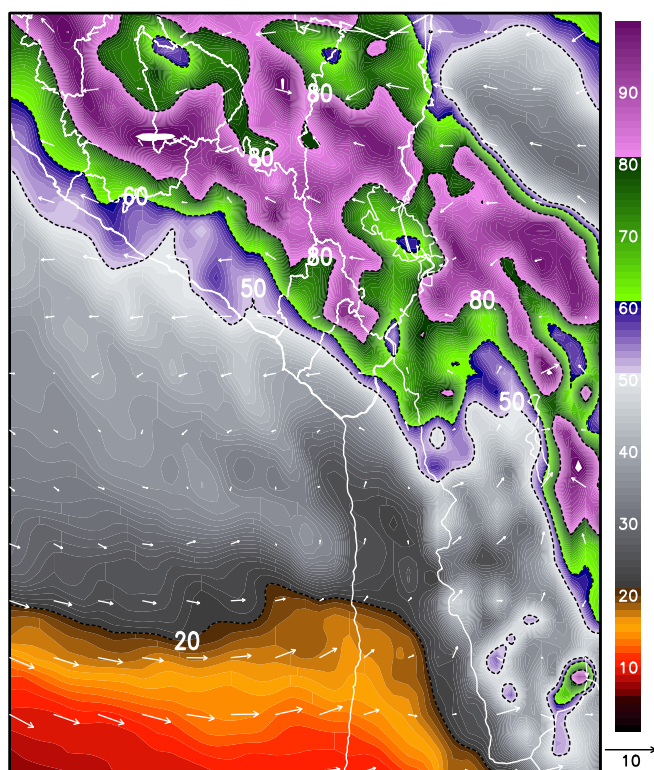
Fig2. Pronóstico de humedad relativa promedio (%) (500-300 hPa) (28/11/2024 – 01:00 pm)
