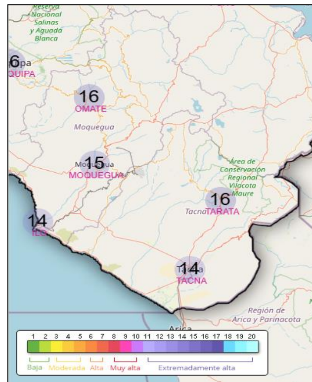
Fig3. Pronóstico de Índice de radiación ultravioleta máximo (IUV) (28/11/2024)
