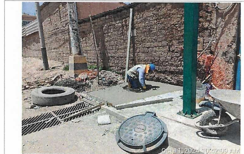
Vaciado de concreto en caja de media tensión eléctrica bocacalle en Óvalo Parque Zonal III, prog. 4+700.
