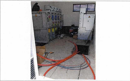
Instalación de celdas Metal Clap en casetas de sub estación.
