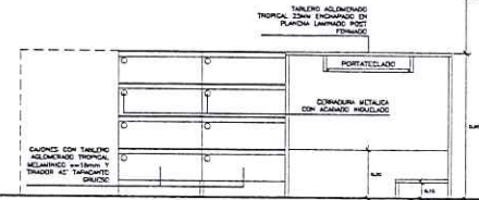
ELEVACIÓN "C" M1 - MUEBLE NUTRICIÓN Y DIETÉTICA ESC. 1/25
