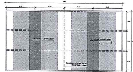
ELEVACIÓN "C" M2 - MUEBLE ALTO DE NUTRICIÓN Y DIETÉTICA ESC. 1/25
