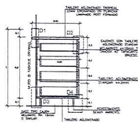
CORTE 2 Mueble Fijo con Cajones ESC. 1/25
