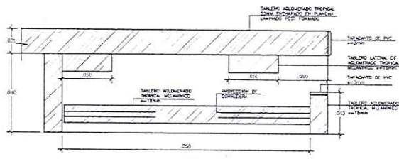
D6 Porta Teclado
