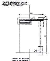
CORTE 1 Mueble Fijo con Portateclado ESC. 1/25
