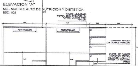
ELEVACIÓN "A" M2 - MUEBLE ALTO DE NUTRICIÓN Y DIETÉTICA ESC. 1/25
