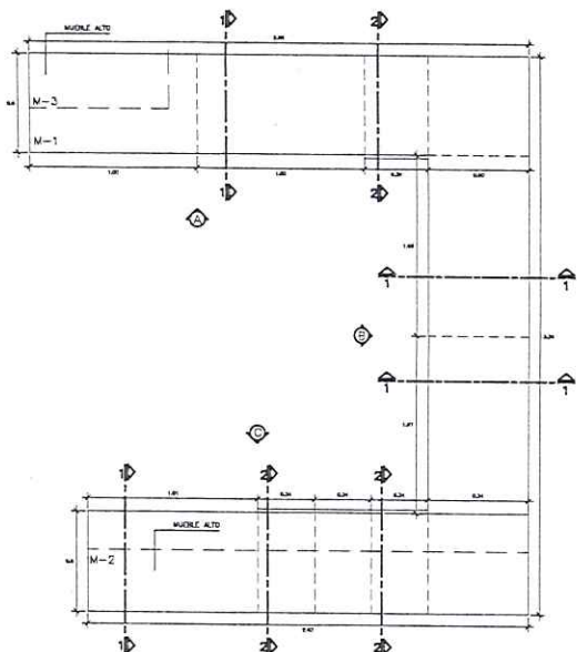
PLANTA M1 - MUEBLE NUTRICIÓN Y DIETÉTICA ESC. 1/25
