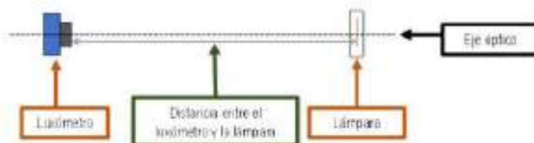
Figura: Esquema de medición de Intensidad Luminosa e Iluminancia.
