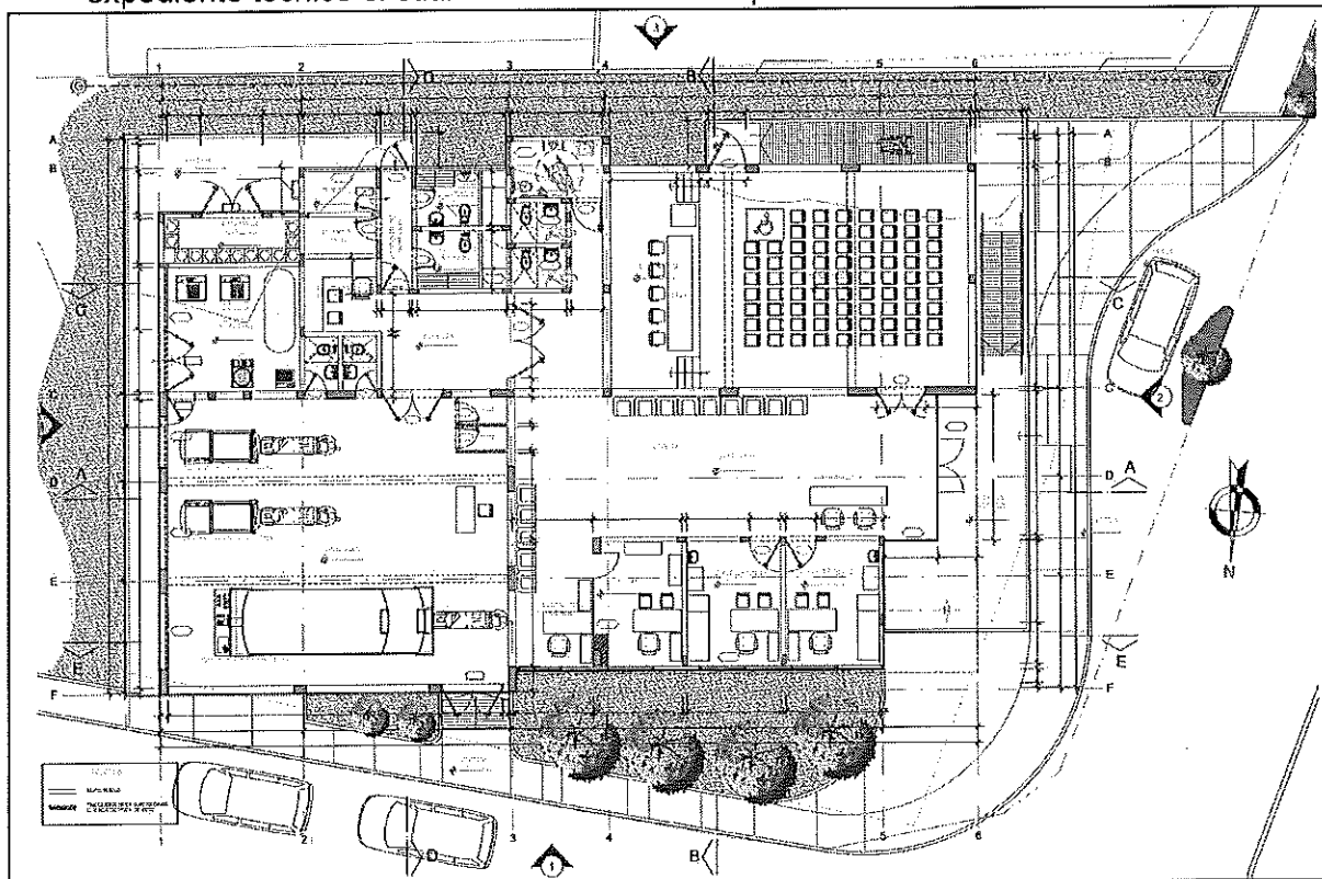
Plano arquitectónico del Proyecto "Creación del Centro de Salud Hiperbárica del Centro Médico Naval en el Distrito de Bellavista"
