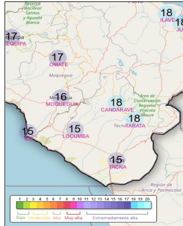
Fig3. Pronóstico de Índice de radiación ultravioleta máximo (IUV) (16/01/2025)
