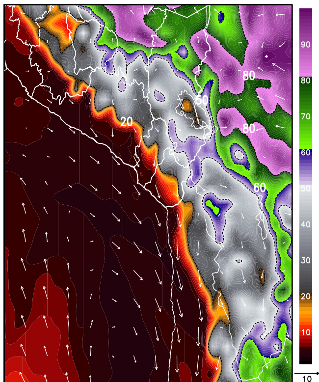
Fig2. Pronóstico de humedad relativa promedio (%) (500-300 hPa) (16/01/2025 – 01:00 pm)
