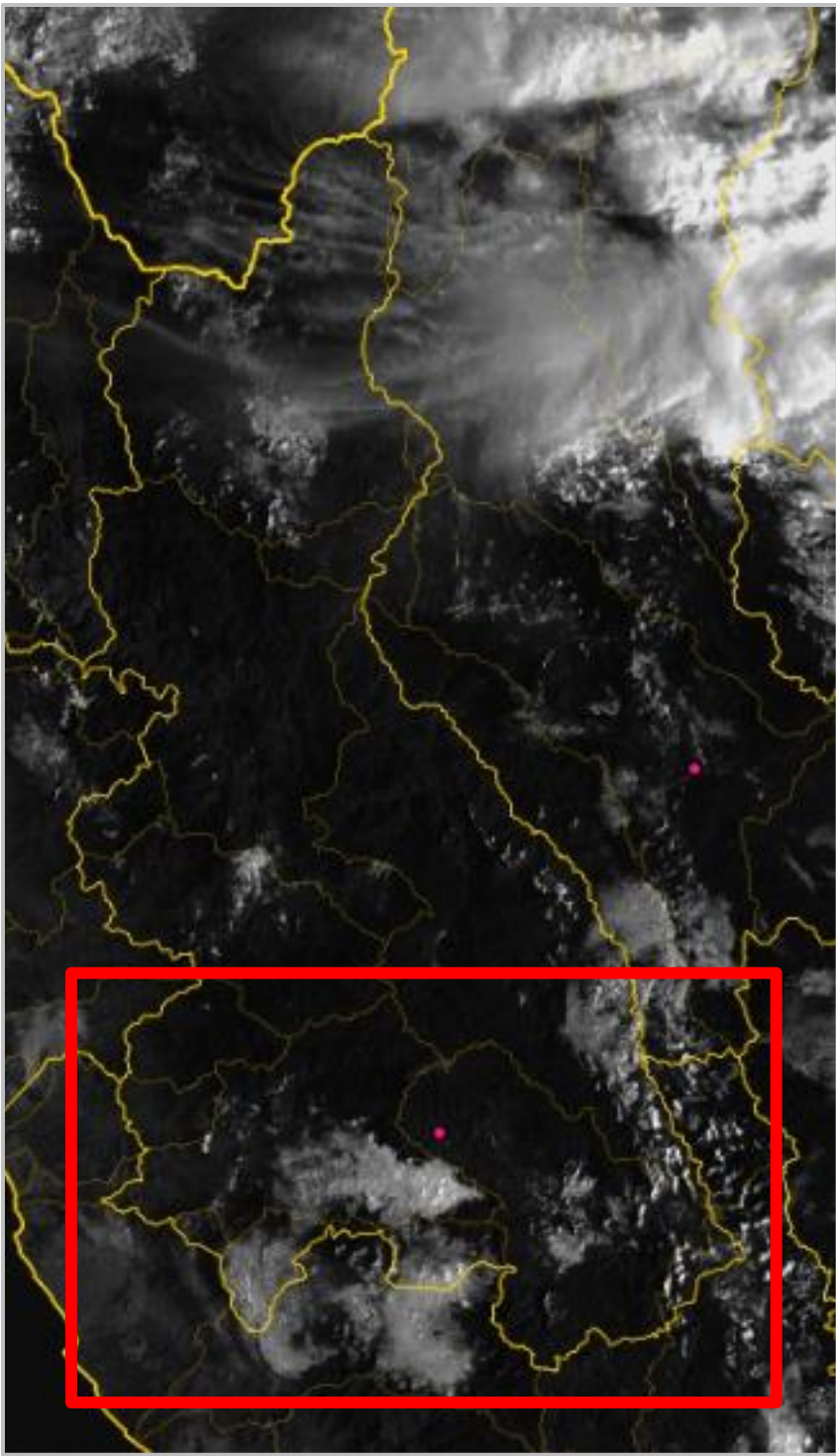
Imagen satelital (rojo) 16/01/2025, 07:30 hora local
