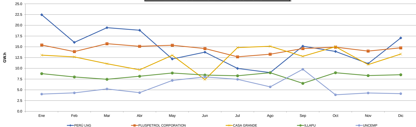
PRODUCCIÓN MENSUAL DE ENERGÍA ELÉCTRICA - ORIGEN TÉRMICO EMPRESAS REPRESENTATIVAS - USO PROPIO
