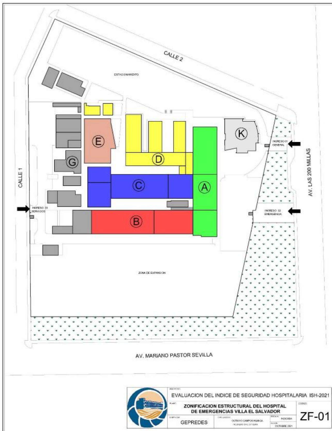
Imagen N° 1. Distribución ARQUITECTÓNICA del Hospital de Emergencias Villa El Salvador
