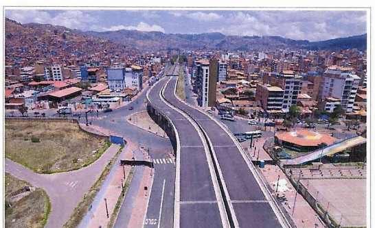
Visualización de la señalización de cruces peatonales. Vista panorámica del Viaducto aéreo - Libertadores (310 m. de longitud). Obra de 6.8 km longitud con 4-vías, 8 carriles, con carpeta asfáltica de e=17 cm en las vías centrales y 13 cm en las vías laterales.
