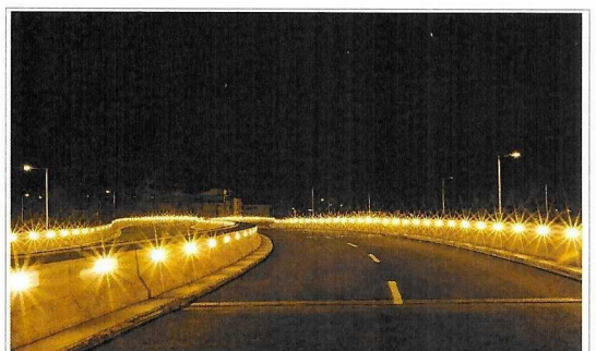
Iluminación vial con lámparas empotradas en los muros new jersey.
