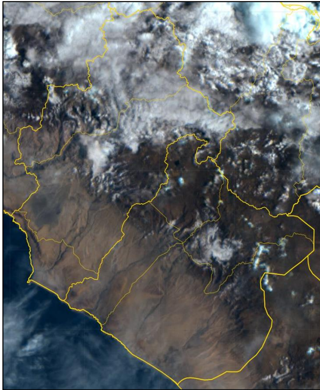
Fig1. Imagen satelital GOES 16 (20/02/2025 – 08:30 am)
