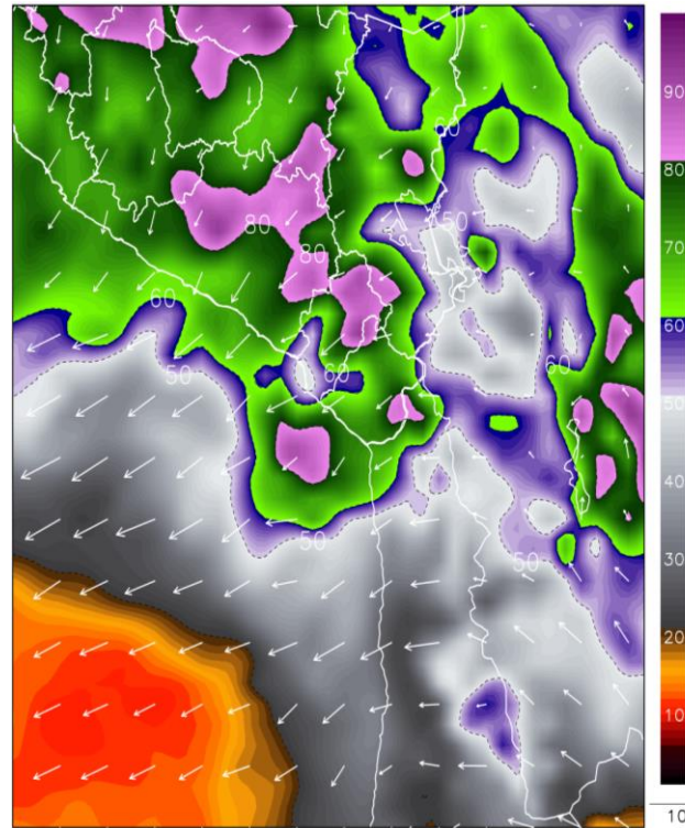
Fig2. Pronóstico de humedad relativa promedio (%) (500-300 hPa) (21/02/2025 – 01:00 pm)
