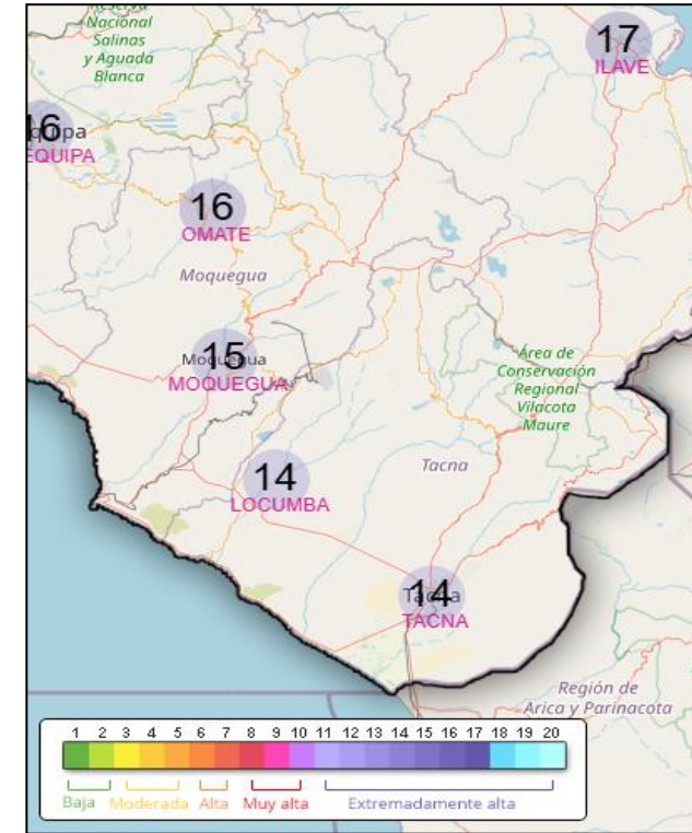
Fig3. Pronóstico de Índice de radiación ultravioleta máximo (IUV) (21/02/2025)
