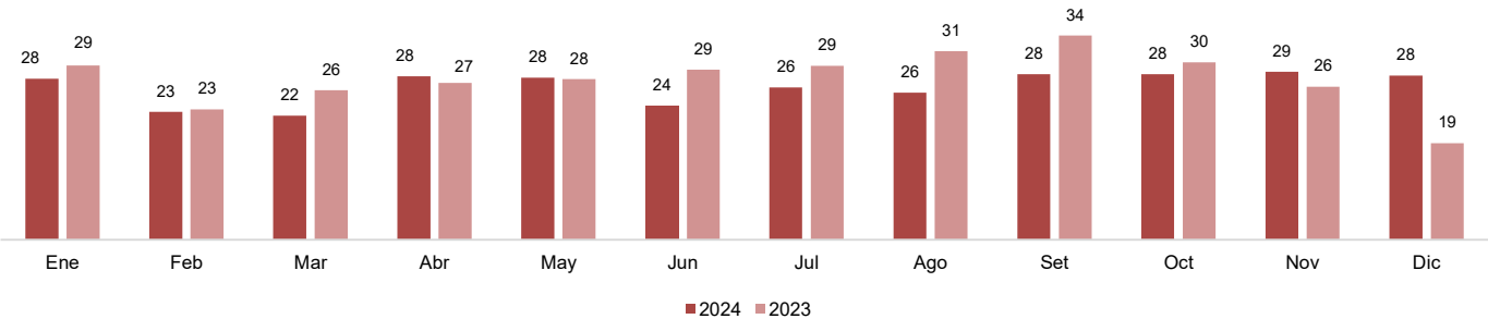
Producción mensual de Cadmio (TMF)
