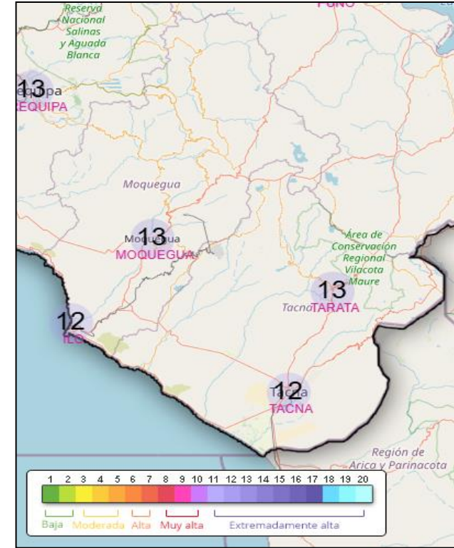
Fig3. Pronóstico de Índice de radiación ultravioleta máximo (IUV) (02/04/2025)
