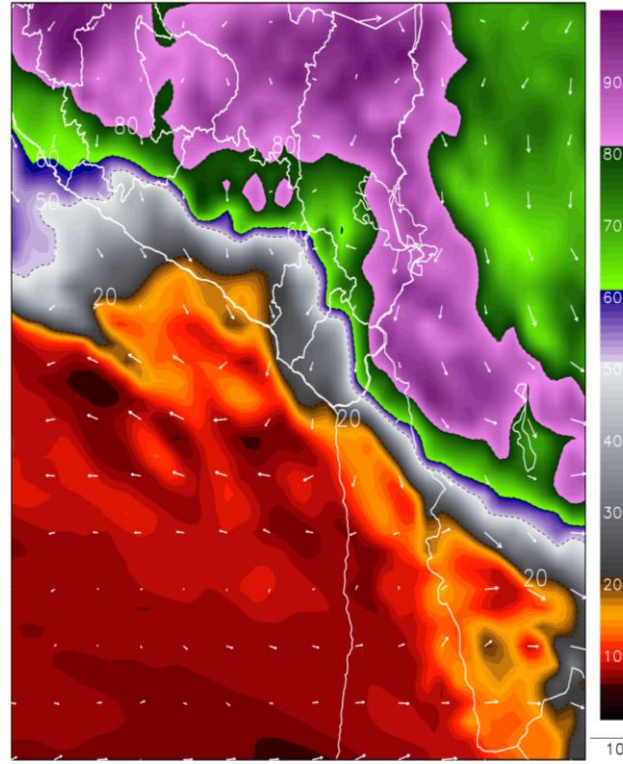
Fig2. Pronóstico de humedad relativa promedio (%) (500-300 hPa) (02/04/2025 – 01:00 pm)
