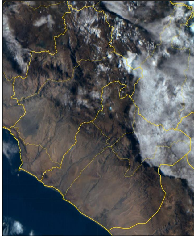
Fig1. Imagen satelital GOES 16 (01/04/2025 – 08:00 am)
