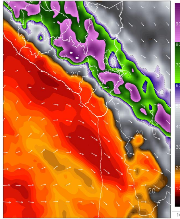
Fig2. Pronóstico de humedad relativa promedio (%) (500-300 hPa) (08/04/2025 – 01:00 pm)
