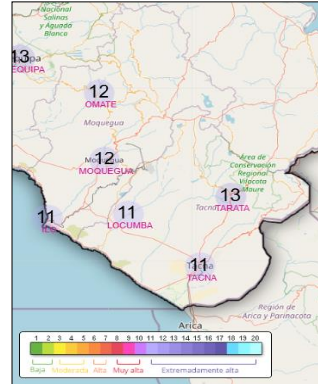
Fig3. Pronóstico de Índice de radiación ultravioleta máximo (IUV) (08/04/2025)
