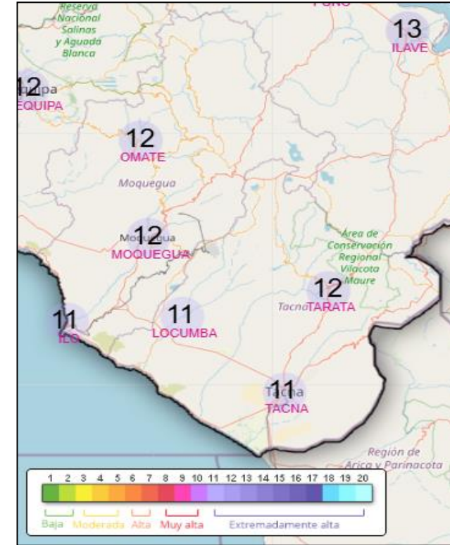
Fig3. Pronóstico de Índice de radiación ultravioleta máximo (IUV) (11/04/2025)
