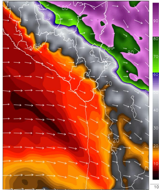
Fig2. Pronóstico de humedad relativa promedio (%) (500-300 hPa) (11/04/2025 – 01:00 pm)
