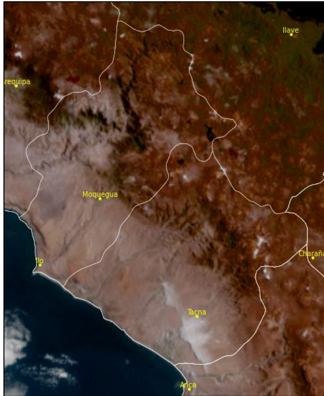
Fig1. Imagen satelital GOES 16 (10/04/2025 – 08:00 am)
