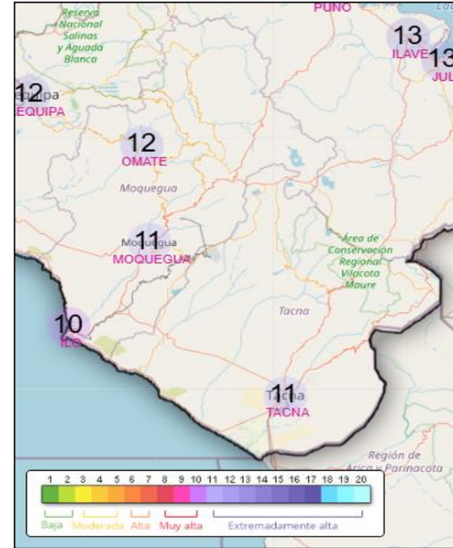
Fig3. Pronóstico de Índice de radiación ultravioleta máximo (IUV) (12/04/2025)
