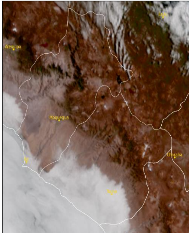
Fig1. Imagen satelital GOES 16 (11/04/2025 – 08:00 am)
