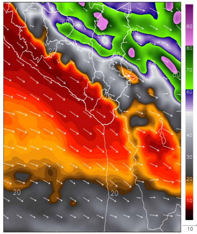
Fig2. Pronóstico de humedad relativa promedio (%) (500-300 hPa) (12/04/2025 – 01:00 pm)
