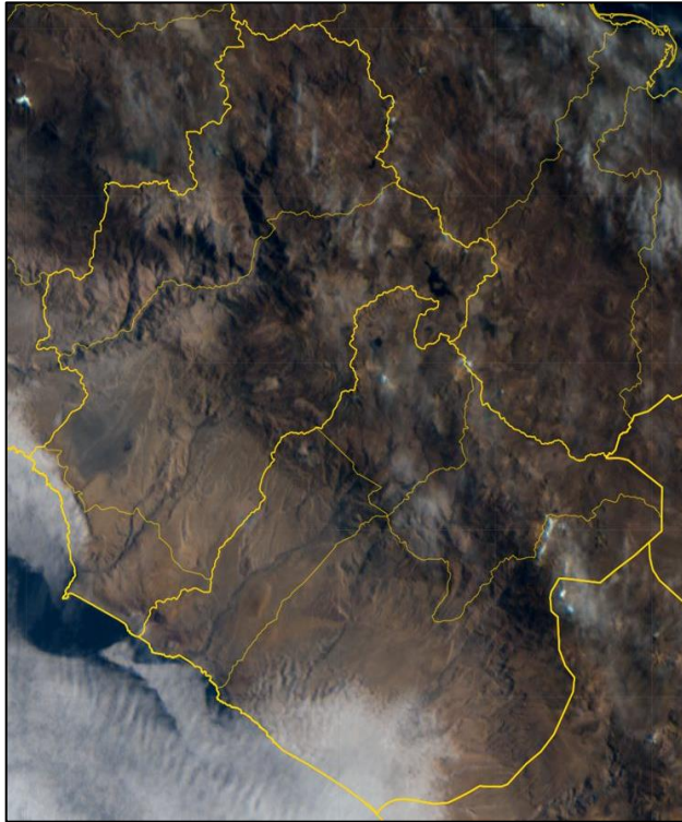
Fig1. Imagen satelital GOES 16 (15/04/2025 – 08:00 am)
