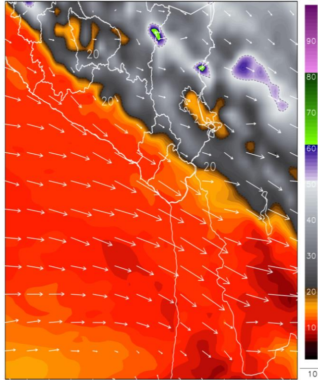
Fig2. Pronóstico de humedad relativa promedio (%) (500-300 hPa) (16/04/2025 – 01:00 pm)
