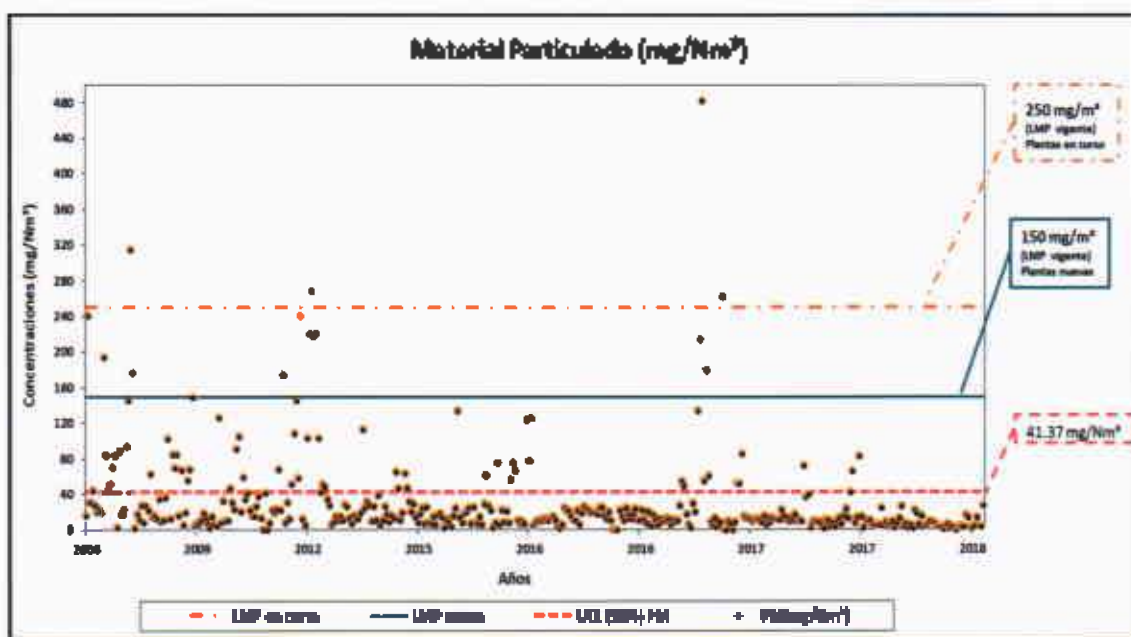
Figura 24: Distribución del conjunto de datos de monitoreo de material particulado
