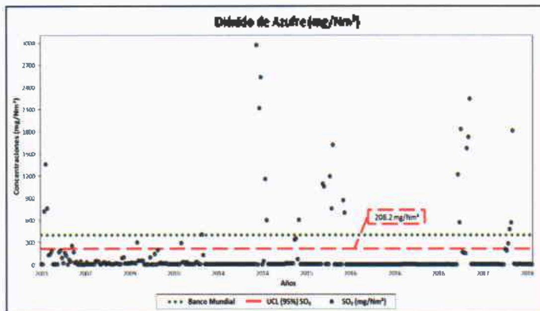
Figura 25: Distribución del conjunto de datos de monitoreo de dióxido de azufre
