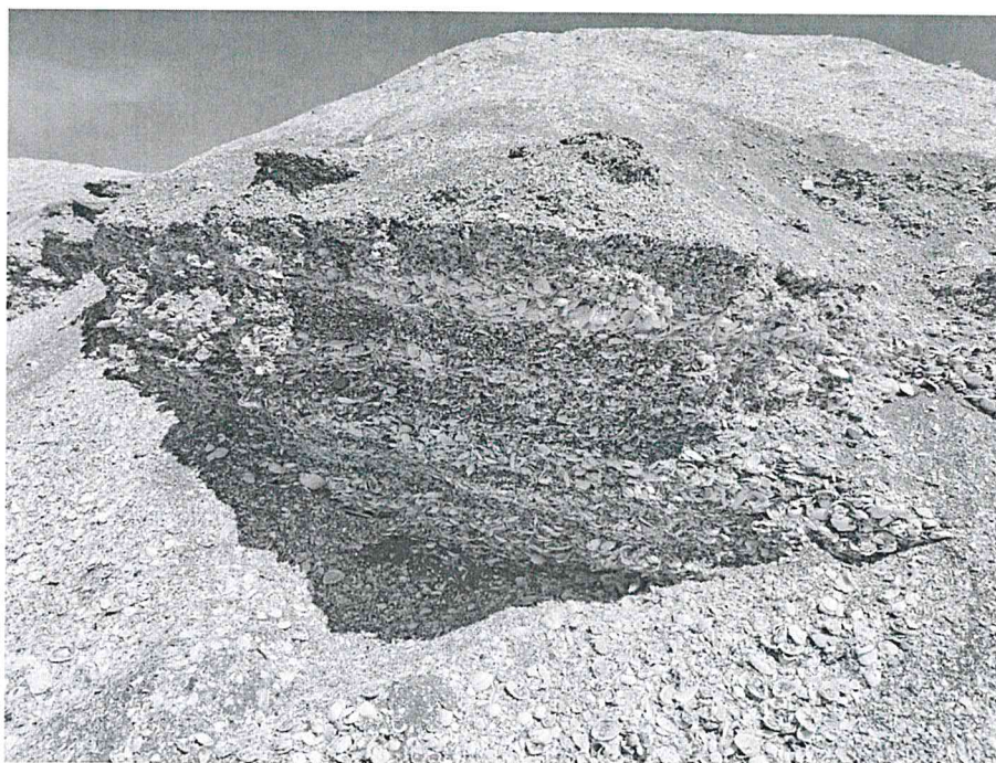
fotografía 9: vista de acumulación de conchales, mostrando el detalle del perfil estratigráfico expuesto, donde se observa los diferentes niveles de ocupación
