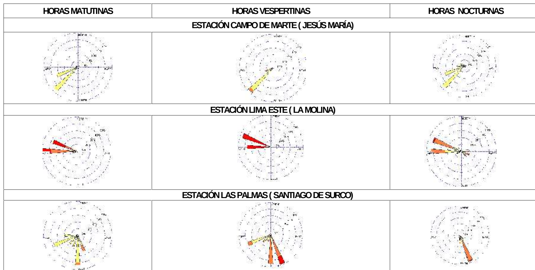
Fig6b – Rosas de viento (m/s) en las estaciones de Jesús María, La Molina y Surco - Noviembre 2007
