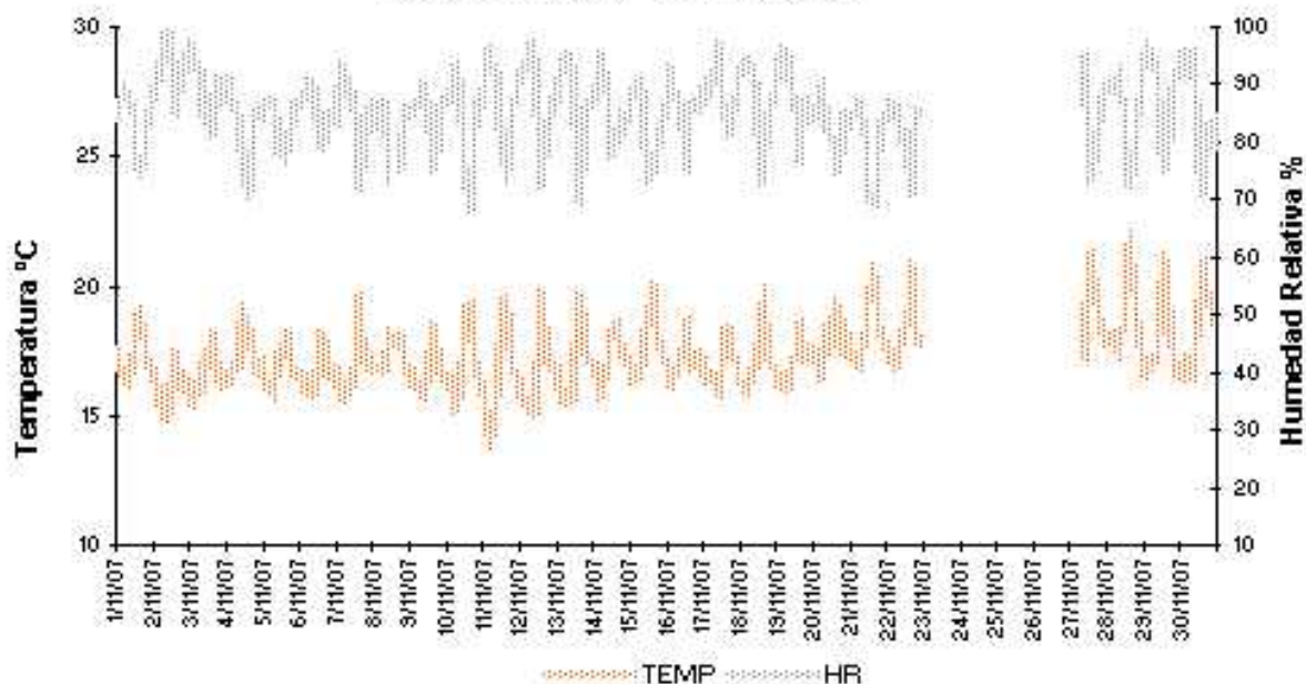
Temperatura y Humedad Relativa Horaria Estacion ANCON - Noviembre 2007
