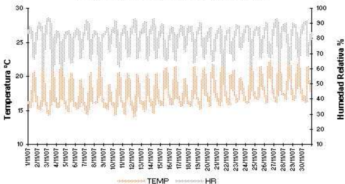
Temperatura y Humedad Relativa Horaria Estacion COLLIQUE (Comas) - Noviembre 2007
