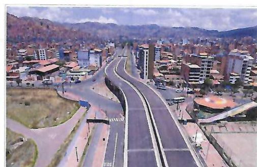
Visualización de la señalización de cruces peatonales. Vista panorámica del Viaducto aéreo - Libertadores (310 m. de longitud) Obra de 6.8 km longitud con 4 vías, 8 carriles, con carpeta asfáltica de e=17 cm en las vías centrales y 13 cm en las vías laterales.
