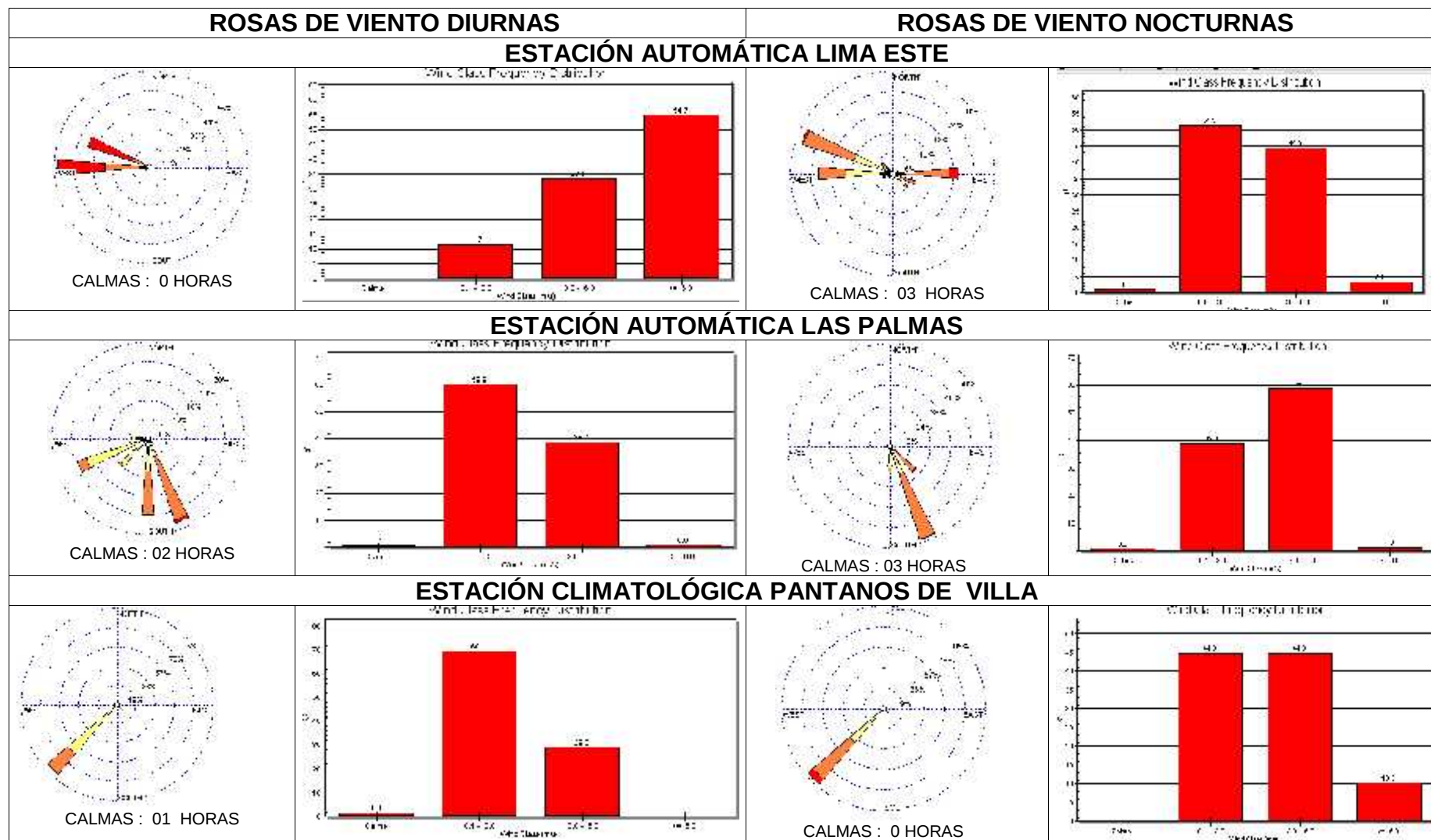
Fig.5b – Rosas de viento (m/s) e histogramas de frecuencia diurnas de las estaciones de La Molina, Santiago de Surco y Chorrillos - Diciembre 2006
