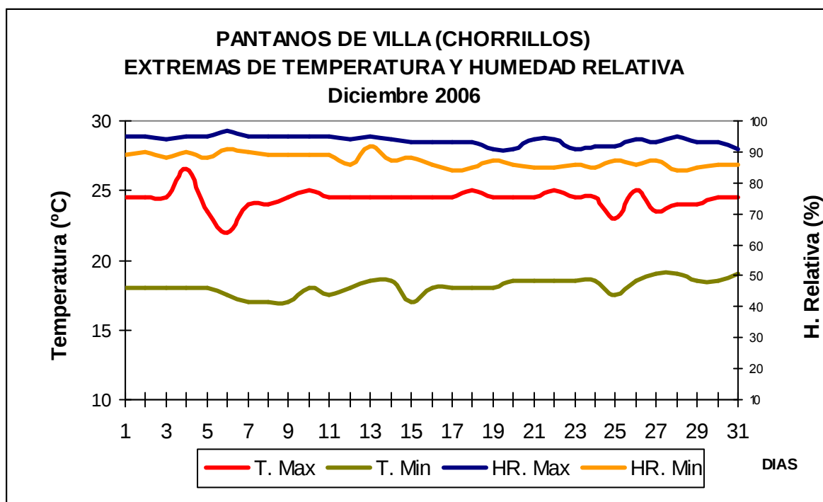
Fig.4- Variación diaria de la temperatura y humedad relativa durante el mes de diciembre del 2006
