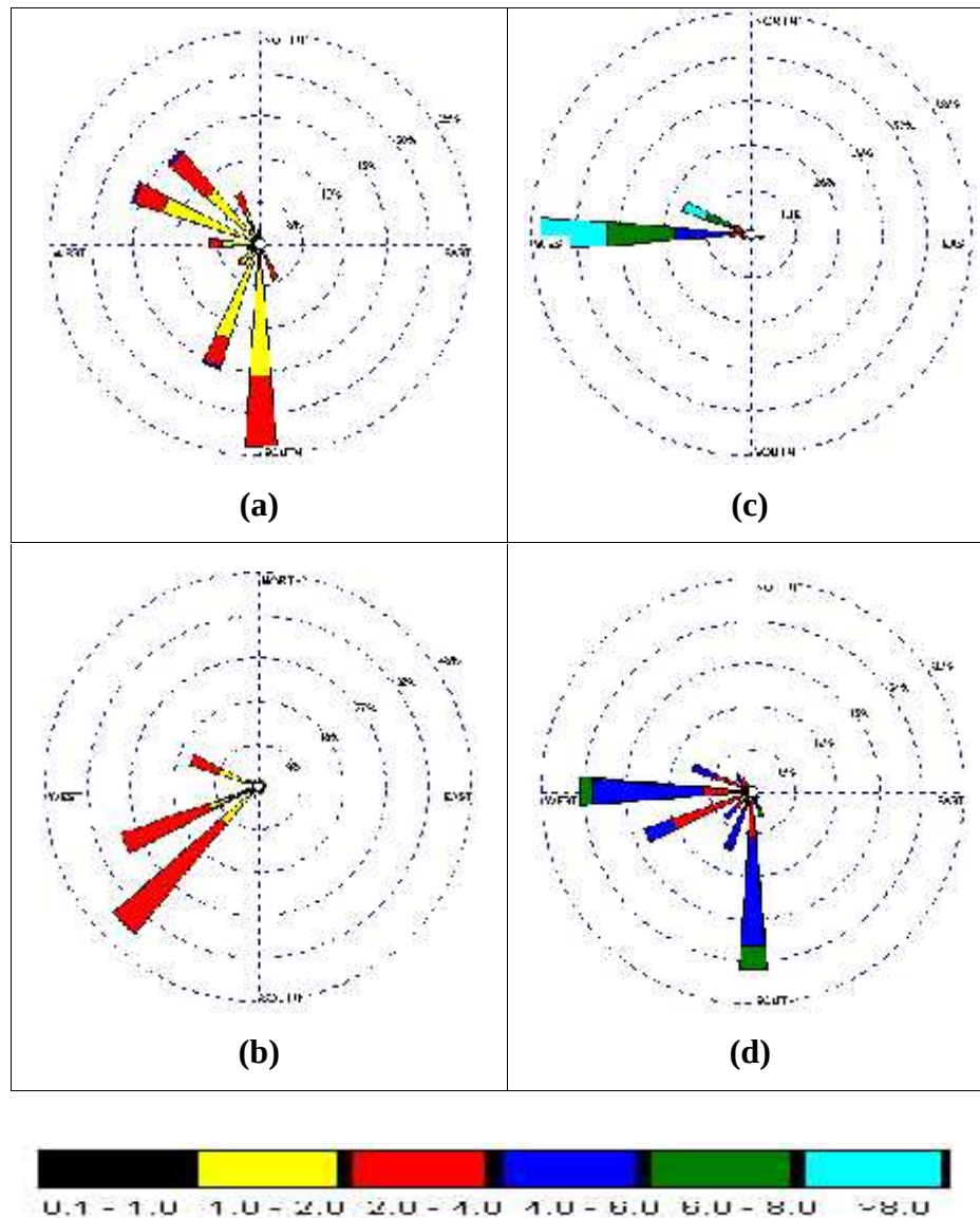
Fig. 6 – Rosas de viento (m/s) diurnas de las estaciones de (a) Jorge Chávez, (b) El Cercado, (c) Lima Este y (d) Las Palmas
