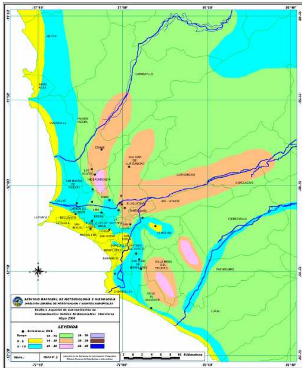
Fig.3 - Distribución espacial de la concentración de sólidos sedimentables en Lima-Callao durante el mes de Mayo del 2004
