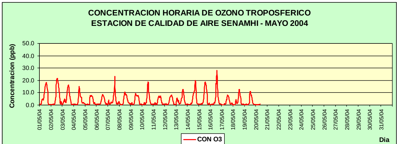
Fig. 4a – Variación temporal de la concentración de Ozono Troposférico durante el mes de Mayo del 2004
