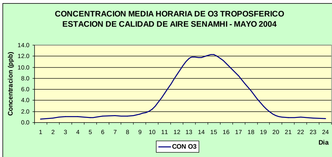
Fig. 4c – Variación media horaria de la concentración de Ozono Troposférico - mes de Mayo del 2004
