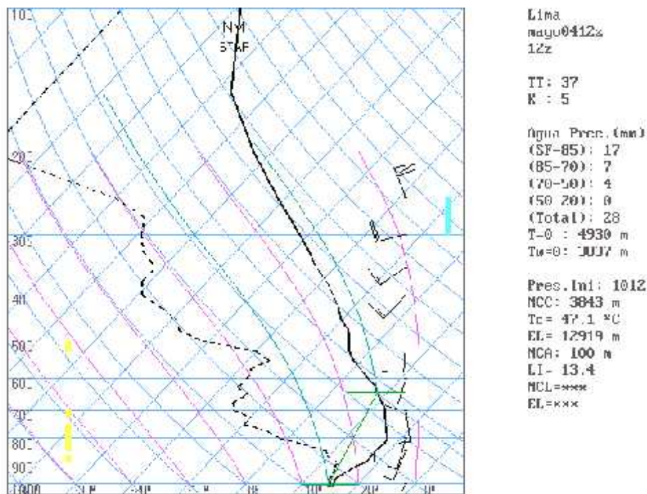
Fig. 8. - Radiosondaje mensual promedio durante el mes de Mayo del 2004 (Aeropuerto Internacional Jorge Chávez)
