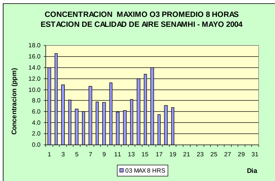
Fig. 4b Variación máxima cada 8 horas de la concentración de Ozono Troposférico - mes de Mayo del 2004
