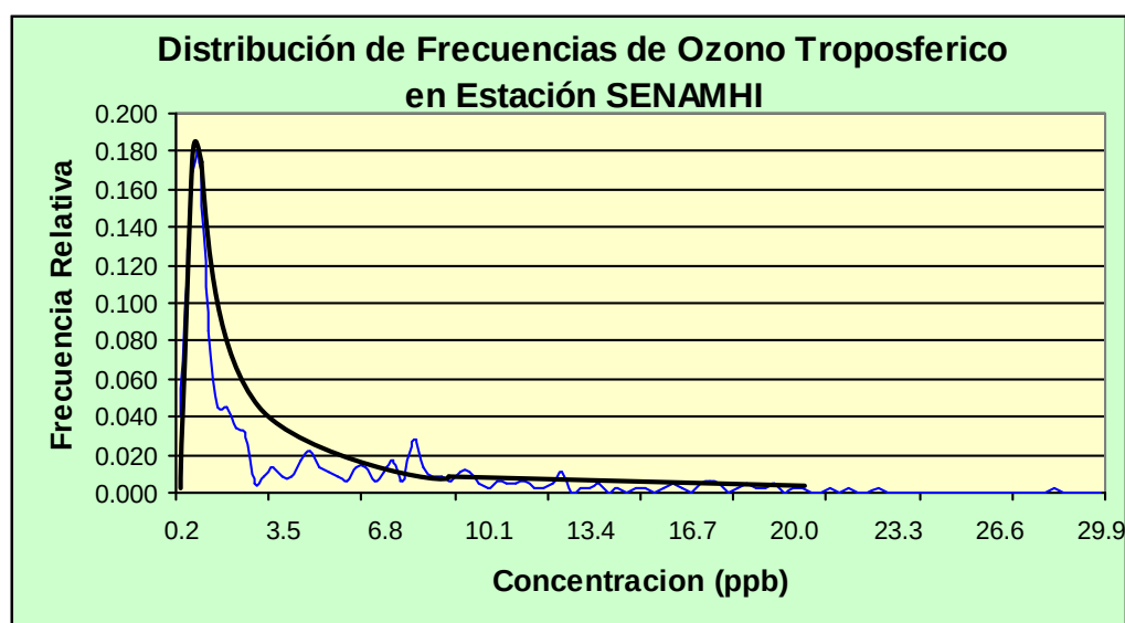
Fig 4d Distribución log-normal de observaciones de Ozono Troposférico
