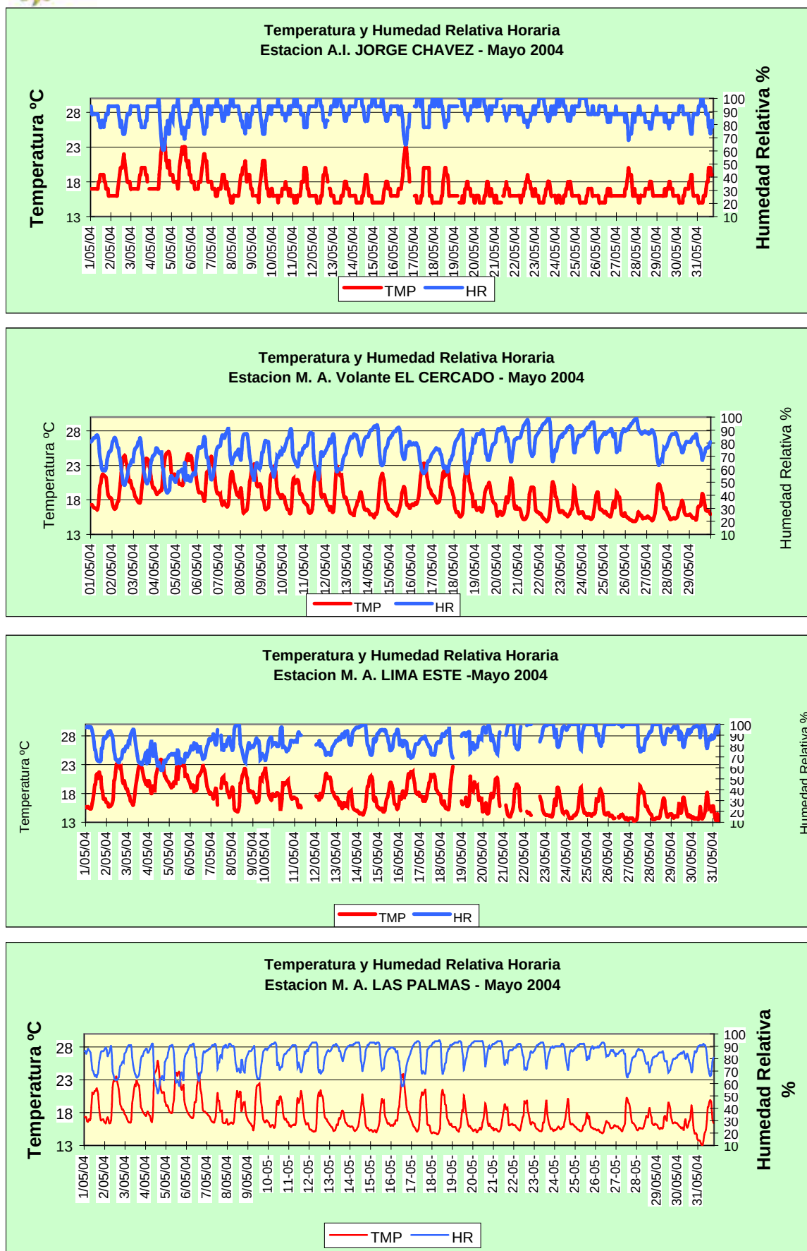
Fig. 5.- Variación horaria de la temperatura y humedad relativa durante el mes de Mayo del 2004 en Lima-Callao
