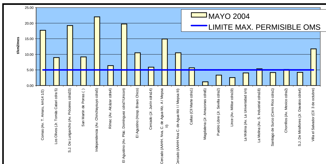
Fig. 2 - Totales mensuales de contaminantes sólidos sedimentables registrados durante el mes de Mayo 2004 en Lima-Callao
