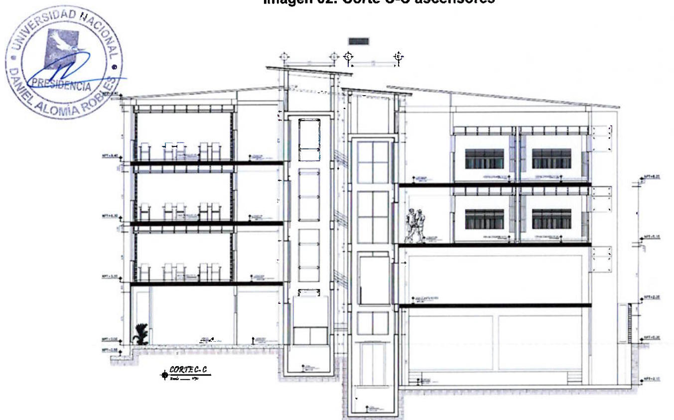
Imagen 02: Corte C-C ascensores
