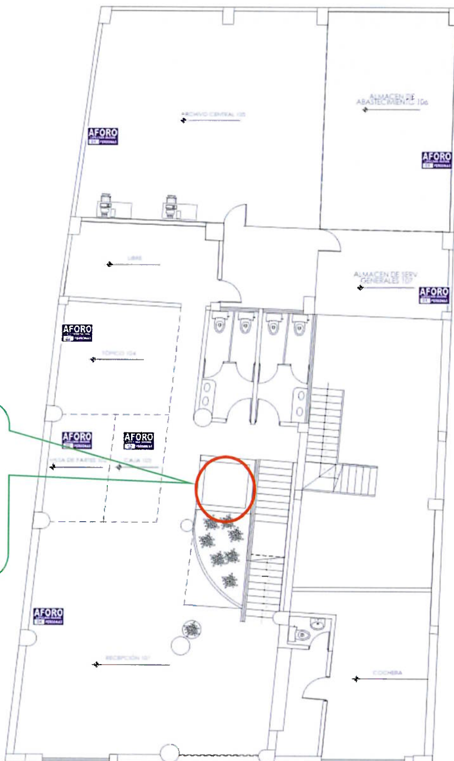
Imagen 19: Plano de Distribución – 1er. Piso
