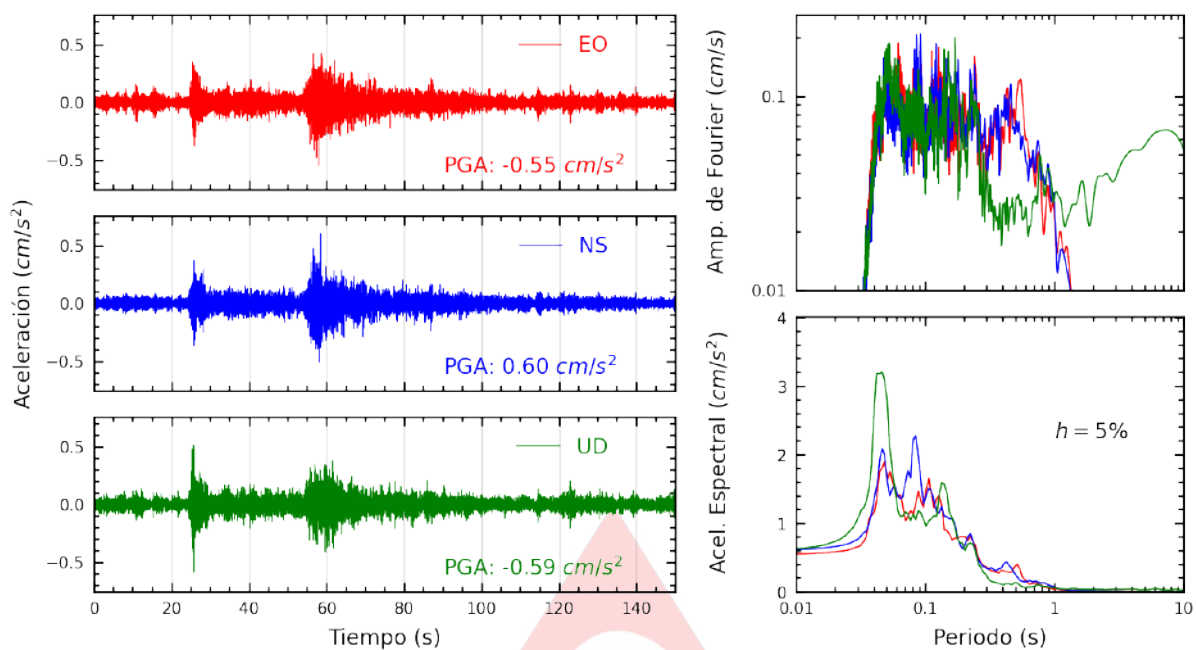
Figura A.1: Registros tiempo-historia, espectros de Fourier y de respuesta en las direcciones EO, NS y UD de la estación SCARQ. Sismo de Calana, Tacna - Tacna de 2025-02-01, 15:27:24 (Hora local)
