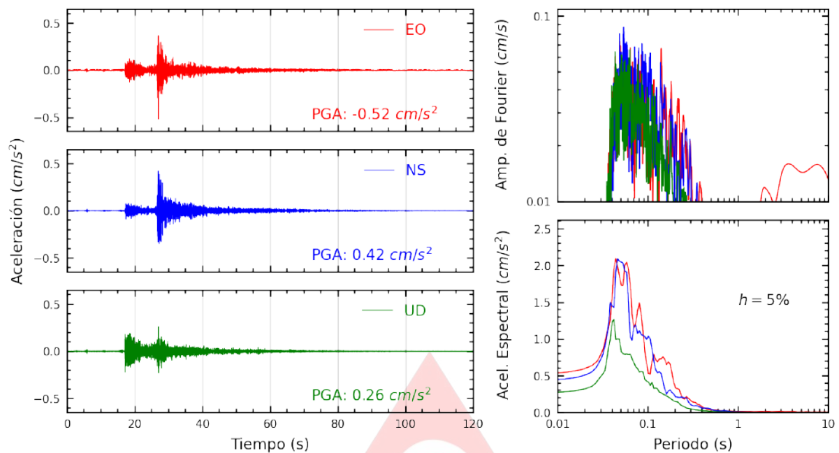
Figura A.1: Registros tiempo-historia, espectros de Fourier y de respuesta en las direcciones EO, NS y UD de la estación SCCHI. Sismo de Olmos, Lambayeque - Lambayeque de 2025-02-02, 01:47:03 (Hora local)
