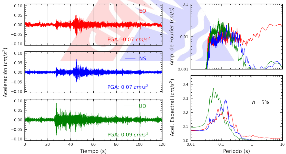
Figura A.2: Registros tiempo-historia, espectros de Fourier y de respuesta en las direcciones EO, NS y UD de la estación SCPIU. Sismo de Olmos, Lambayeque - Lambayeque de 2025-02-02, 01:47:03 (Hora local)
