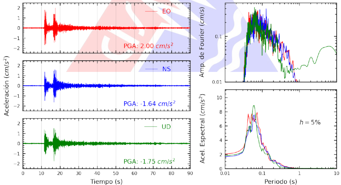
Figura A.2: Registros tiempo-historia, espectros de Fourier y de respuesta en las direcciones EO, NS y UD de la estación SCARQ. Sismo de La Capilla, General Sanchez Cerro - Moquegua de 2025-02-08, 15:42:04 (Hora local)
