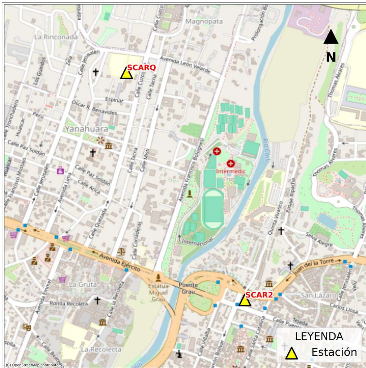
Figura 2: Mapa de ubicación de la(s) estación(es) acelerográfica(s) que registraron el Sismo de La Capilla, General Sanchez Cerro - Moquegua del 08 de febrero de 2025 a las 15:42:04 (hora local)
