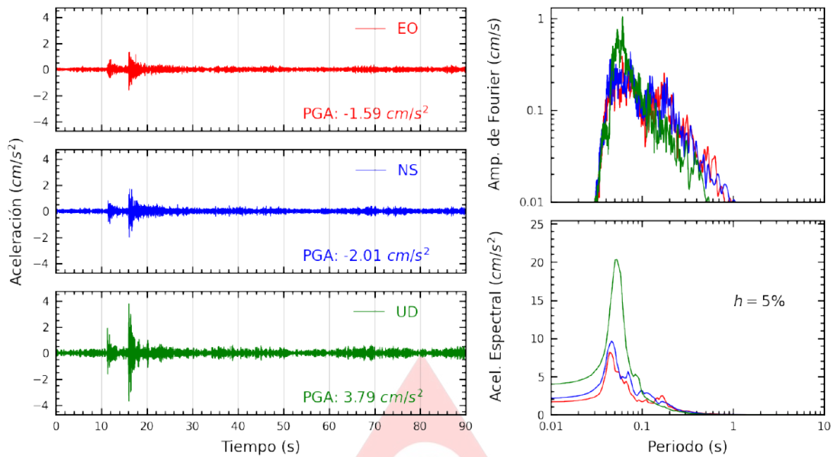
Figura A.1: Registros tiempo-historia, espectros de Fourier y de respuesta en las direcciones EO, NS y UD de la estación SCAR2. Sismo de La Capilla, General Sanchez Cerro - Moquegua de 2025-02-08, 15:42:04 (Hora local)
