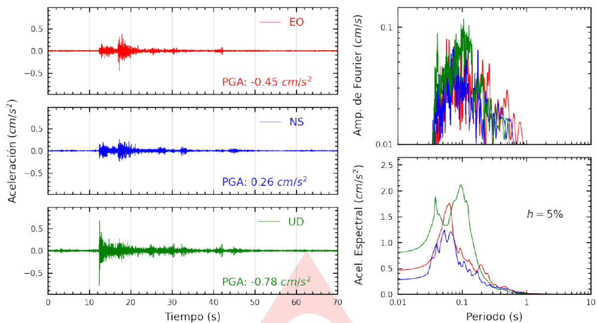
Figura A.1: Registros tiempo-historia, espectros de Fourier y de respuesta en las direcciones EO, NS y UD de la estación SCCUS. Sismo de Paruro, Paruro - Cusco de 2025-02-08, 05:23:45 (Hora local)
