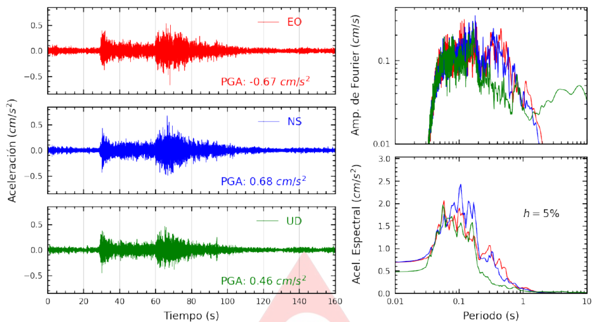
Figura A.1: Registros tiempo-historia, espectros de Fourier y de respuesta en las direcciones EO, NS y UD de la estación SCARQ. Sismo de Tacna, Tacna - Tacna de 2025-02-10, 21:00:27 (Hora local)
