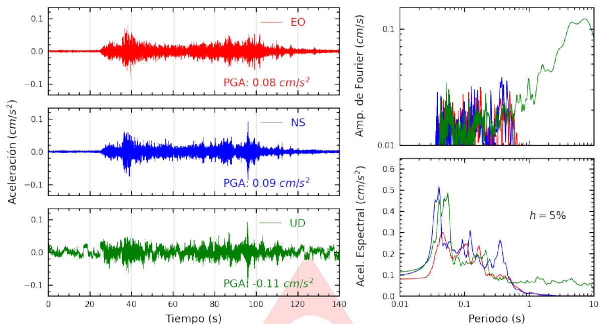
Figura A.1: Registros tiempo-historia, espectros de Fourier y de respuesta en las direcciones EO, NS y UD de la estación SCARQ. Sismo de Cabanaconde, Caylloma - Arequipa de 2025-02-12, 01:32:08 (Hora local)
