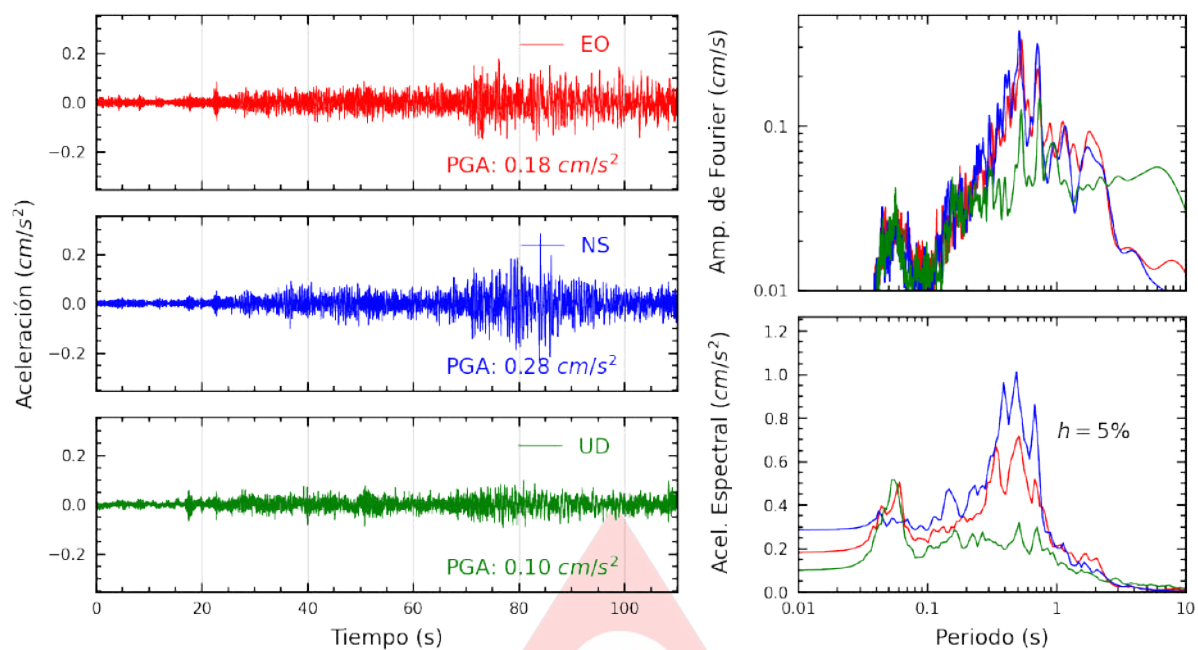
Figura A.1: Registros tiempo-historia, espectros de Fourier y de respuesta en las direcciones EO, NS y UD de la estación SCARQ. Sismo de Lomas, Caraveli - Arequipa de 2025-02-16, 23:30:54 (Hora local)
