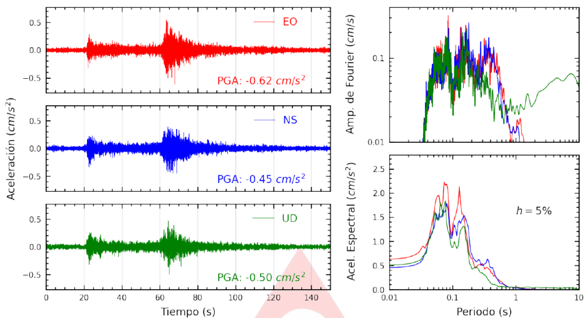
Figura A.1: Registros tiempo-historia, espectros de Fourier y de respuesta en las direcciones EO, NS y UD de la estación SCARQ. Sismo de Tacna, Tacna - Tacna de 2025-02-16, 16:00:56 (Hora local)
