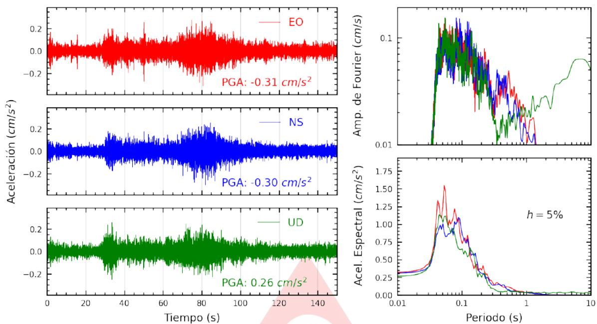
Figura A.1: Registros tiempo-historia, espectros de Fourier y de respuesta en las direcciones EO, NS y UD de la estación SCARQ. Sismo de Ilave, El Collao - Puno de 2025-02-17, 11:34:09 (Hora local)
