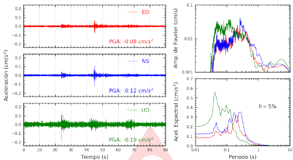
Figura A.1: Registros tiempo-historia, espectros de Fourier y de respuesta en las direcciones EO, NS y UD de la estación SCPUC. Sismo de Pampa Hermosa, Ucayali - Loreto de 2025-02-17, 08:33:16 (Hora local)
