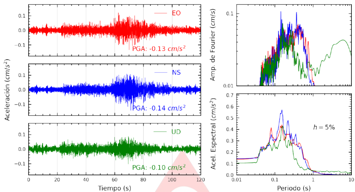
Figura A.1: Registros tiempo-historia, espectros de Fourier y de respuesta en las direcciones EO, NS y UD de la estación SCARQ. Sismo de Yauca, Caraveli - Arequipa de 2025-02-17, 01:04:03 (Hora local)
