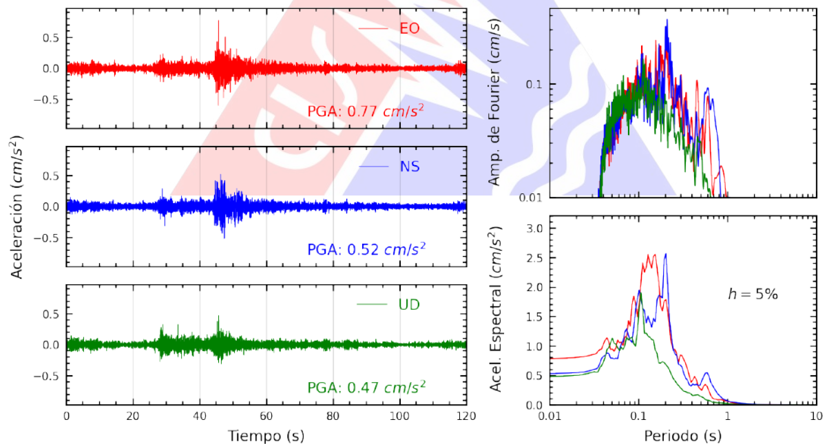
Figura A.2: Registros tiempo-historia, espectros de Fourier y de respuesta en las direcciones EO, NS y UD de la estación SCCHO. Sismo de Canta, Canta - Lima de 2025-02-20, 21:03:25 (Hora local)
