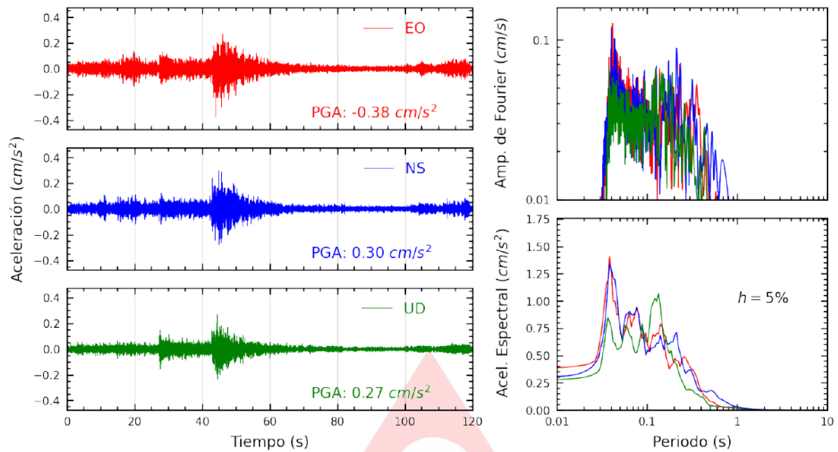
Figura A.1: Registros tiempo-historia, espectros de Fourier y de respuesta en las direcciones EO, NS y UD de la estación BORJA. Sismo de Canta, Canta - Lima de 2025-02-20, 21:03:25 (Hora local)
