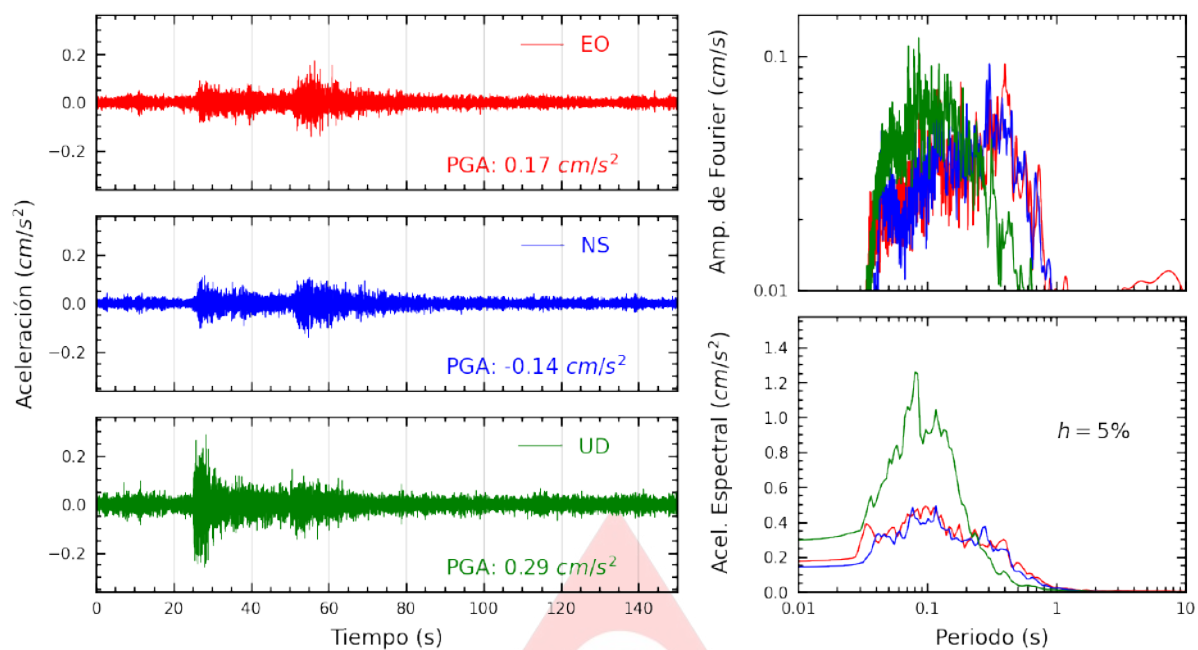
Figura A.1: Registros tiempo-historia, espectros de Fourier y de respuesta en las direcciones EO, NS y UD de la estación SCPIU. Sismo de Ayabaca, Ayabaca - Piura de 2025-02-21, 17:52:09 (Hora local)
